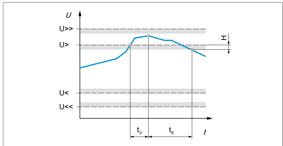
Rysunek 53: Monitorowanie napięcia z przykładowym przekroczeniem wartości granicznej Przepięcie U>
