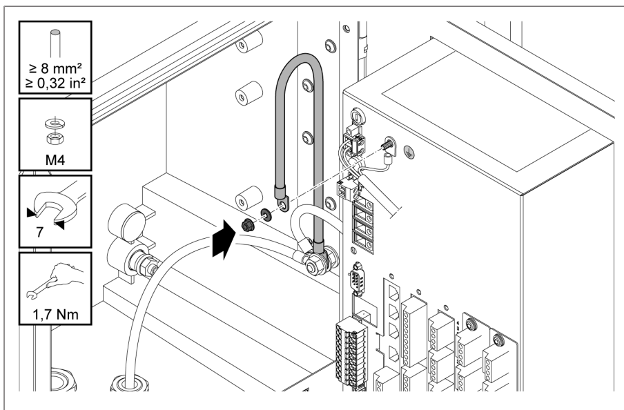
Rysunek 37: Mocowanie kabla uziemiającego obudowy i przewodu ochronnego urządzenia
