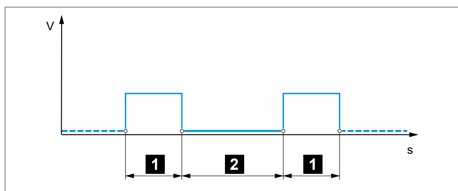
Rysunek 67: Czas trwania impulsu wyzwalającego i przerwa między impulsami wyzwalającymi
