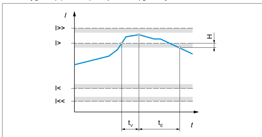
Rysunek 54: Monitorowanie prądu z przykładowym przekroczeniem wartości granicznej I>
