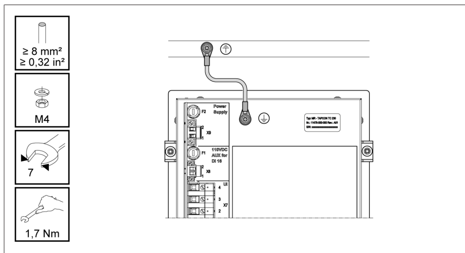
Rysunek 35: Podłączanie kabla uziemiaczego
