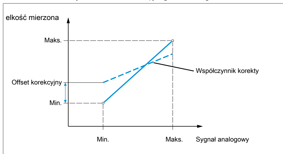
Rysunek 42: Sygnał analogowy z charakterystyką liniową, współczynnik korekty <1 i offset korekcyjny
