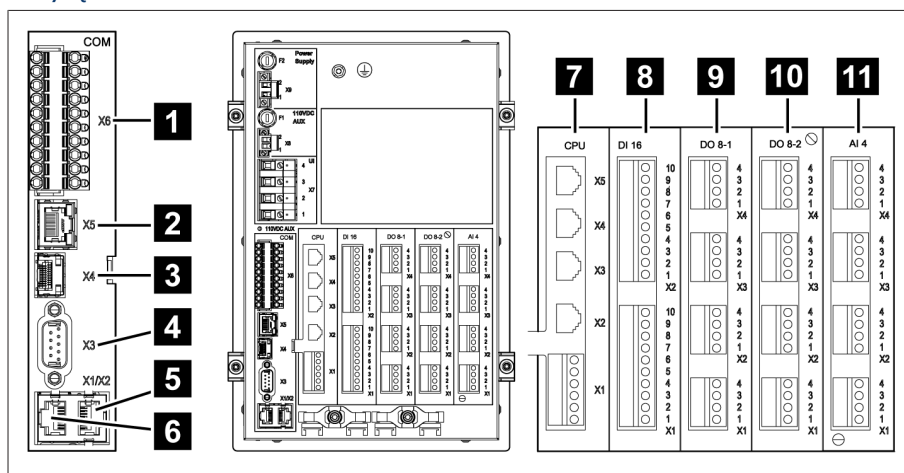
Rysunek 5: Przyłącza/zaciski
