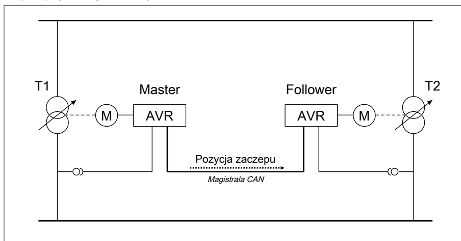
Rysunek 64: Synchronizacja zaczeów
