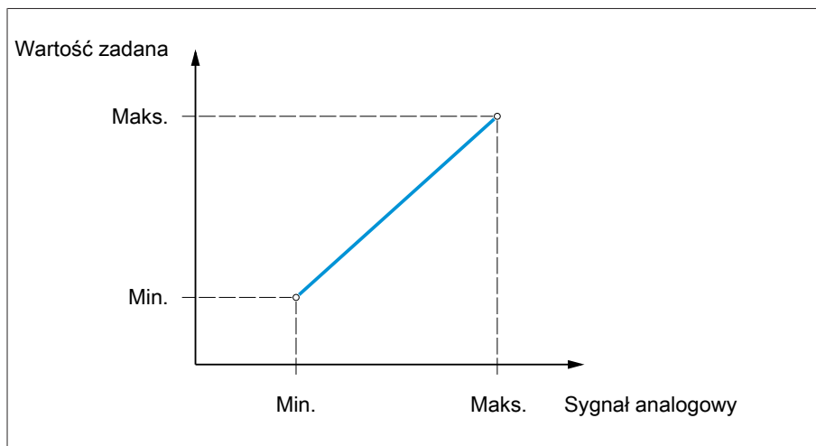
Rysunek 56: Analogowe ustawianie wartości zadanej
