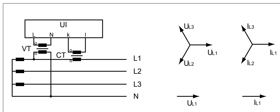
Rysunek 48: Obwód 1-B
