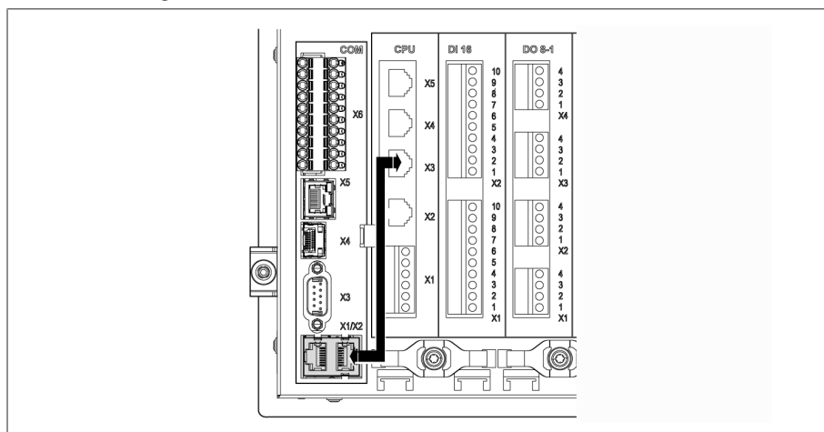
Rysunek 68: Kabel krosowy z tyłu
