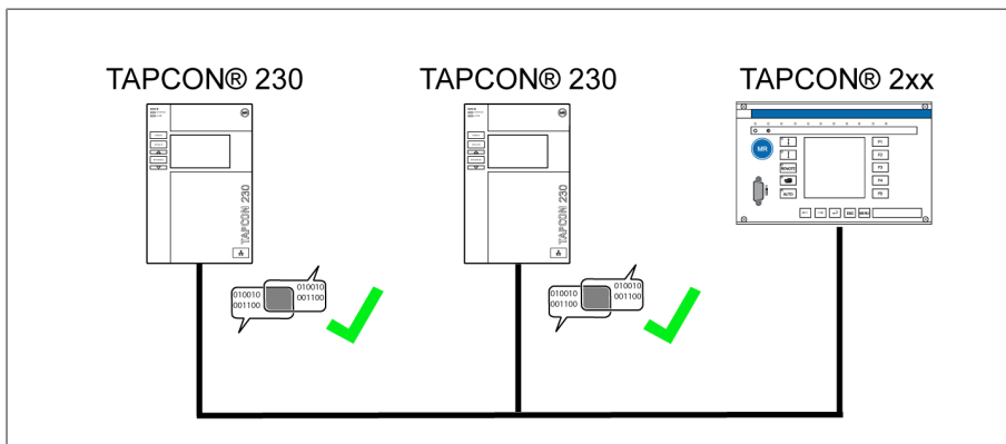
Rysunek 55: Działanie równoległe 2 urządzeń z jednym urządzeniem TAPCON® 2xx
