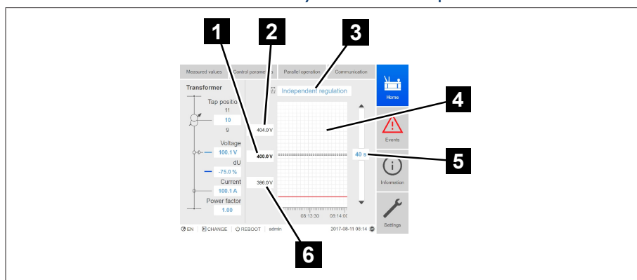
Rysunek 10: Wartości zadane / wartości rzeczywiste / czas opóźnienia
