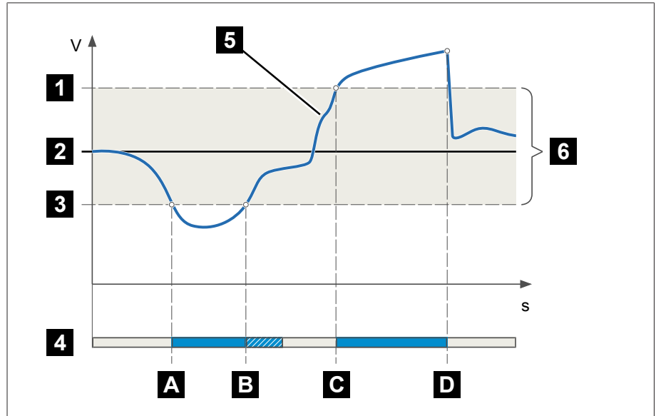
Rysunek 58: Charakterystyka pracy funkcji regulacji z czasem opóźnienia T1
