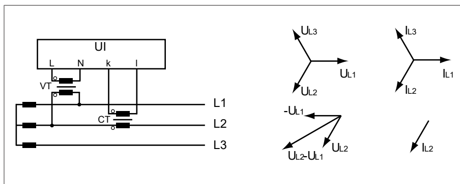
Rysunek 51: Obwód 1-E
