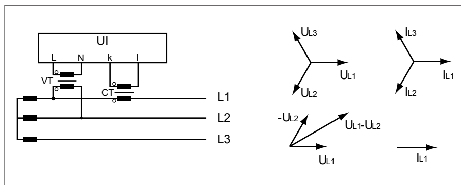
Rysunek 52: Obwód 1-F
