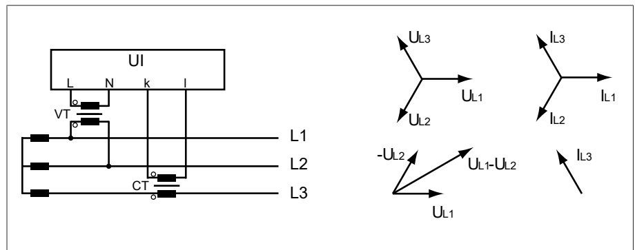
Rysunek 50: Obwód 1-D
