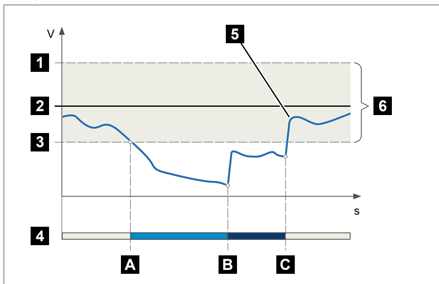
Rysunek 60: Charakterystyka pracy funkcji regulacji z czasem opóźnienia T1 i T2
