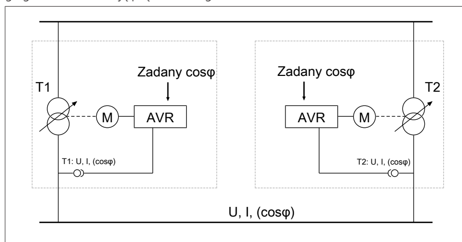
Rysunek 66: Minimalizacja prądu biernego w obwodzie bez komunikacji magistrali CAN
