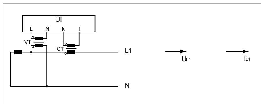
Rysunek 47: Obwód 1-A
