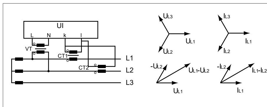
Rysunek 49: Obwód 1-C
