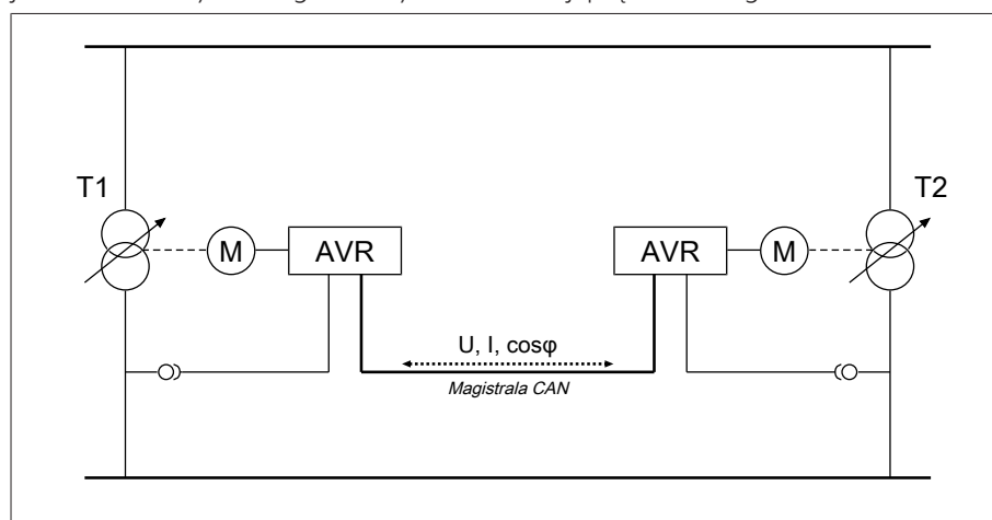
Rysunek 65: Minimalizacja prądu biernego w obwodzie z komunikacją z magistrali CAN
