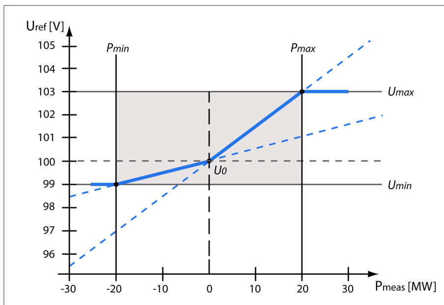
Rysunek 57: Dostosowanie wartości zadanej napięcia uzależnione od mocy czynnej
