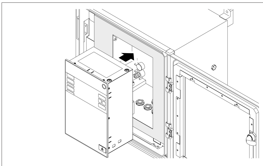
Rysunek 23: Wsuwanie urządzenia w ramę uchylną
