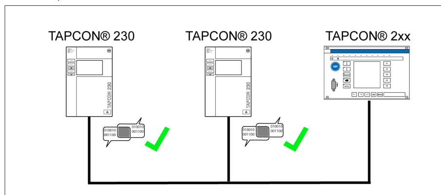
Figura 60: Marcha en paralelo de 2 aparatos con un TAPCON® 2xx
