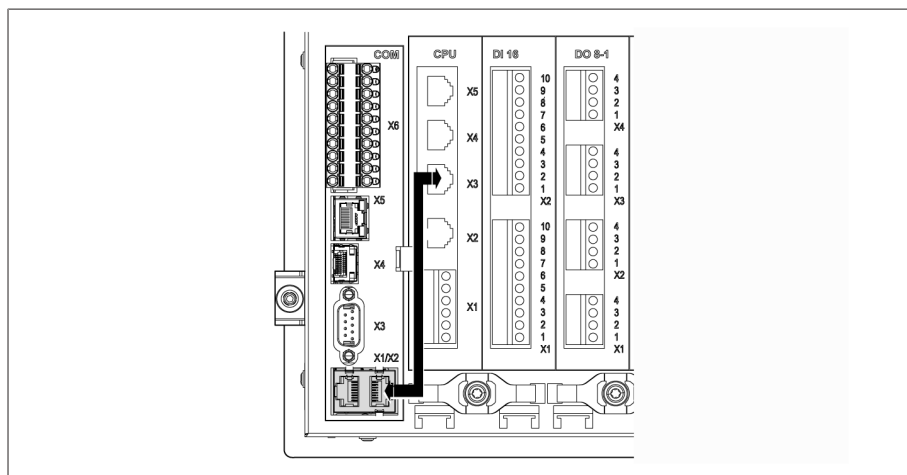
Figura 73: Cable patch en la parte posterior
