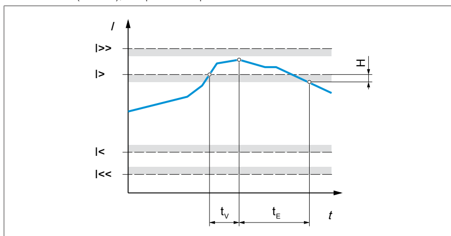
Figura 59: Control de corriente con exceso del valor límite superior I> a modo de ejemplo
