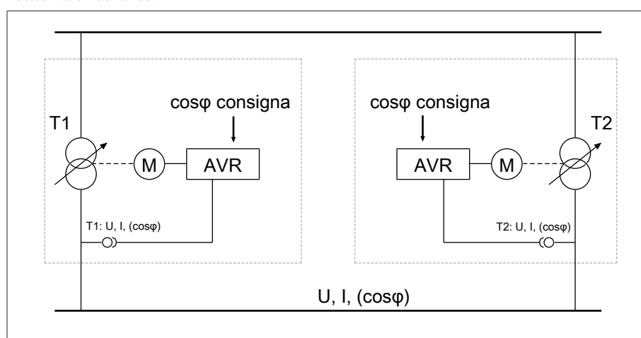
Figura 71: Reducción de la corriente reactiva circulante sin comunicación bus CAN
