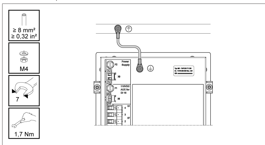
Figura 35: Conexión del cable de puesta a tierra
