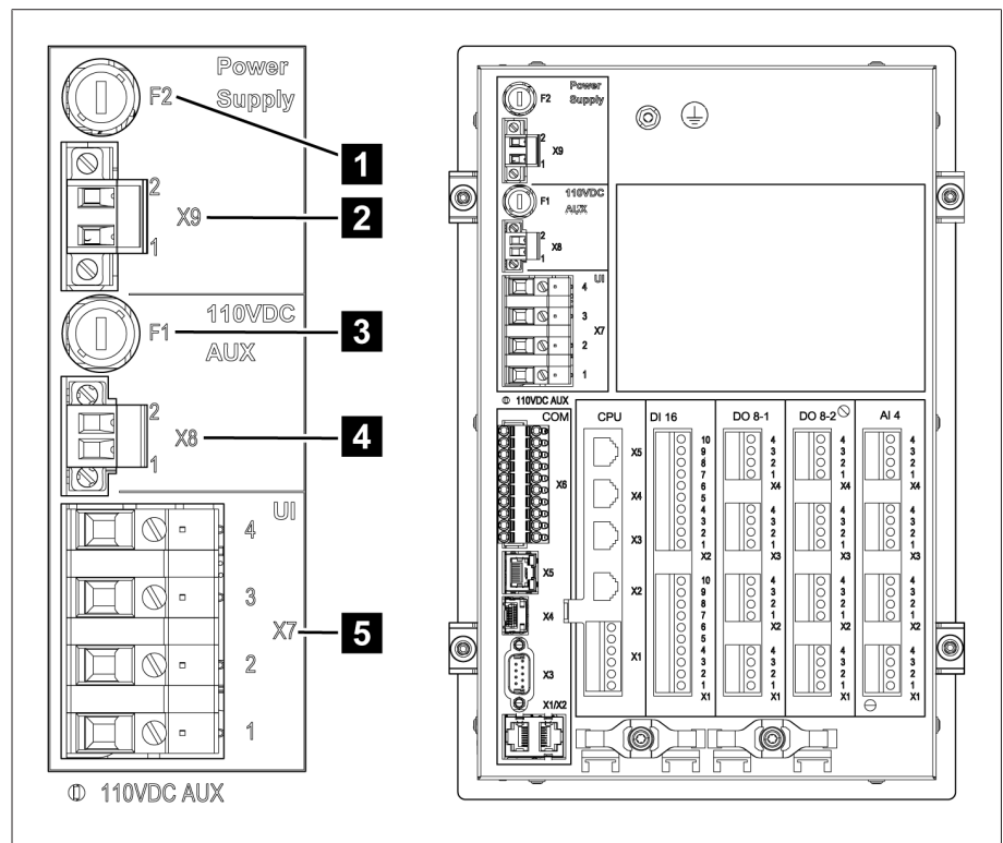
Figura 4: Lado trasero
