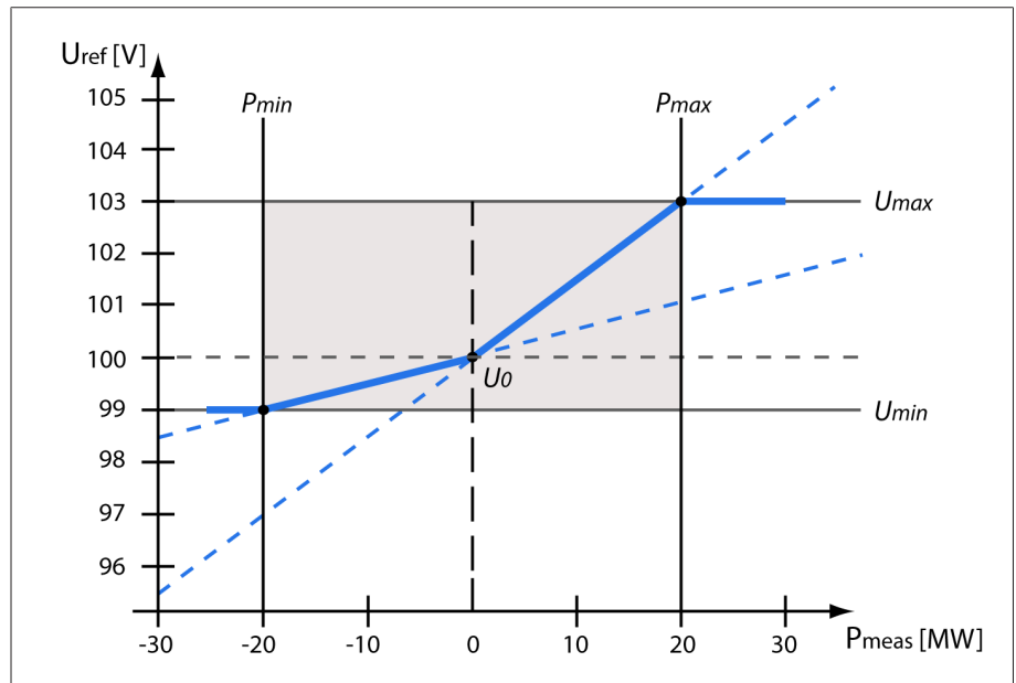
Figura 62: Adaptación del valor consigna de tensión dependiente de la potencia activa
