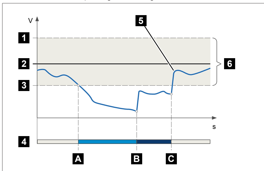
Figura 65: Comportamiento de la función de regulación con tiempo de retardo T1 y T2
