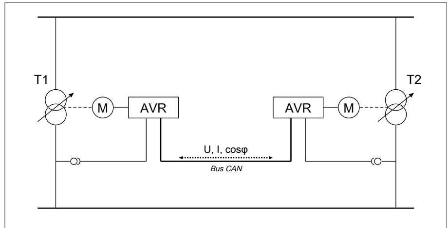
Figura 70: Reducción de la corriente reactiva circulante con comunicación bus CAN
