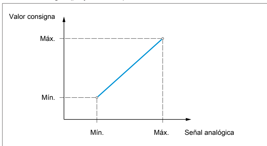
Figura 61: Especificación de valor consigna analógica
