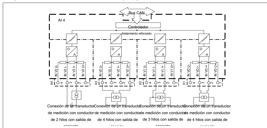
Figura 33: Esquema de conexiones de bloque para entradas analógicas
