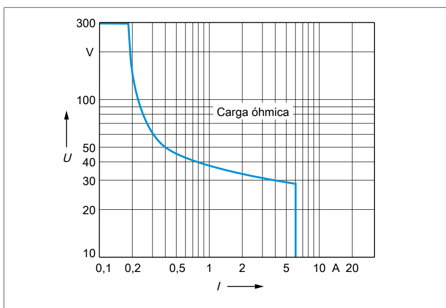
Figura 77: Carga del contacto de las salidas digitales con carga óhmica
