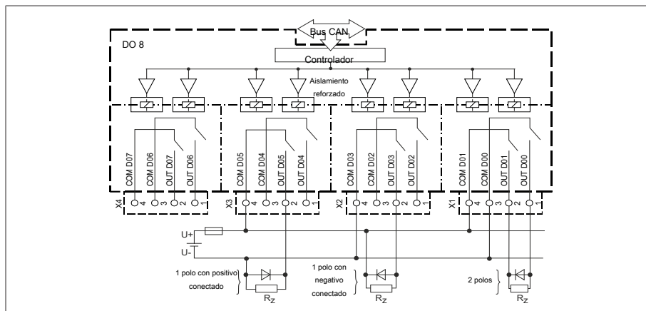
Figura 34: Esquema de conexiones de bloque para salidas digitales
