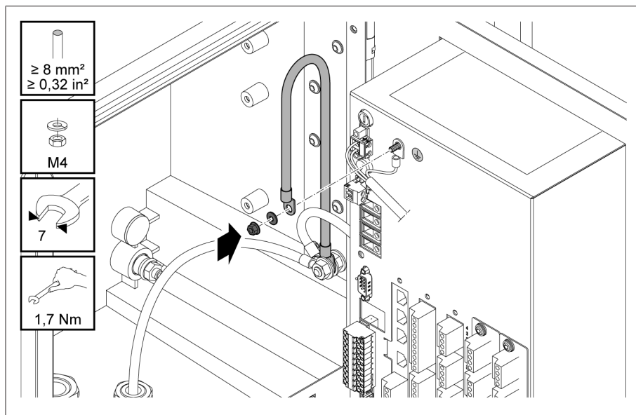
Figura 37: Fijación del cable de puesta a tierra de la carcasa en el conductor de tierra del aparato
