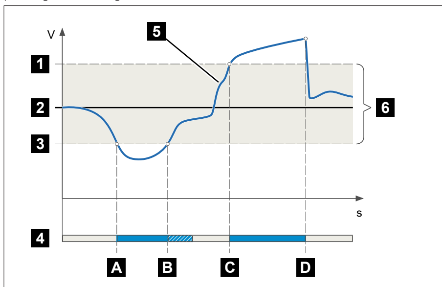
Figura 63: Comportamiento de la función de regulación con tiempo de retardo T1
