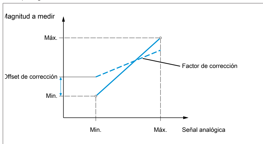
Figura 44: Señal analógica con curva característica lineal, factor de corrección <1 y offset de corrección
