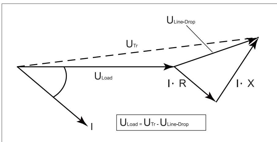
Figura 67: Representación en vectores de la compensación R-X
