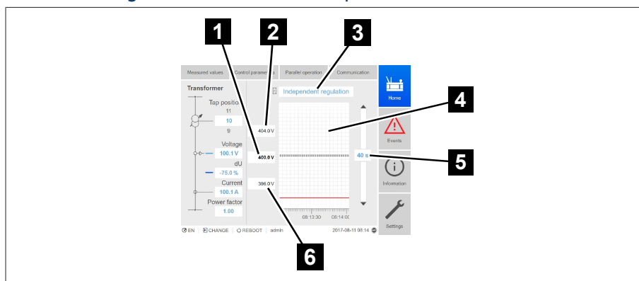
Figura 10: Valores consigna/valores reales/tiempo de retardo
