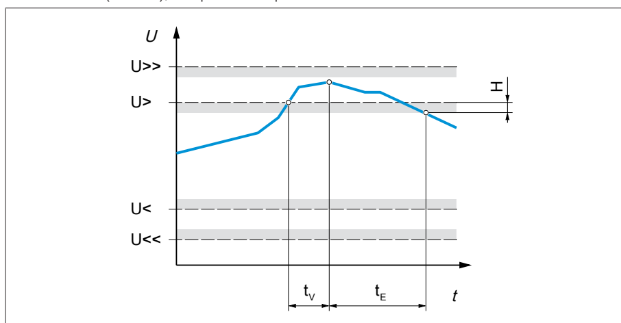
Figura 58: Control de tensión con exceso del valor límite superior Sobre-tensión U>
