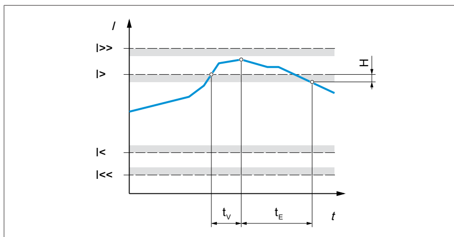
Рис. 51: Контроль тока с примером превышения граничного значения I_{>}
