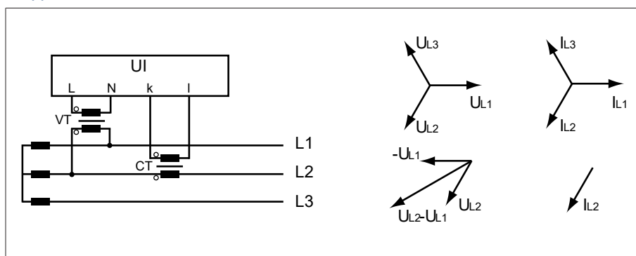
Рис. 48: Подключение 1-E
