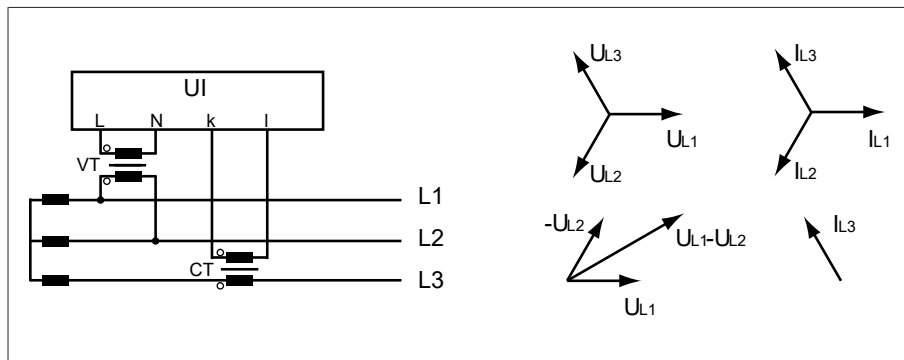
Рис. 47: Подключение 1-D
