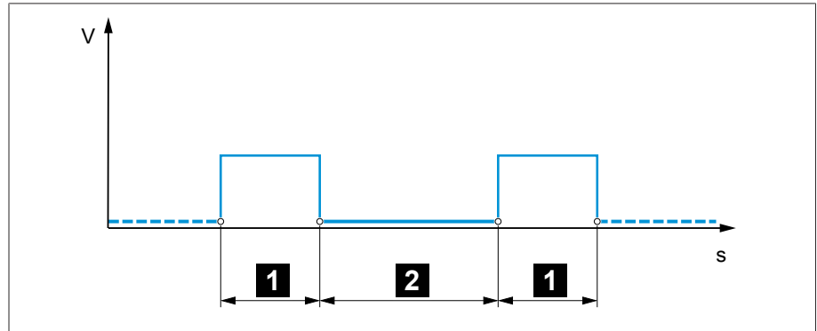
Рис. 59: Длительность управляющего импульса и пауза между управляющими импульсами
