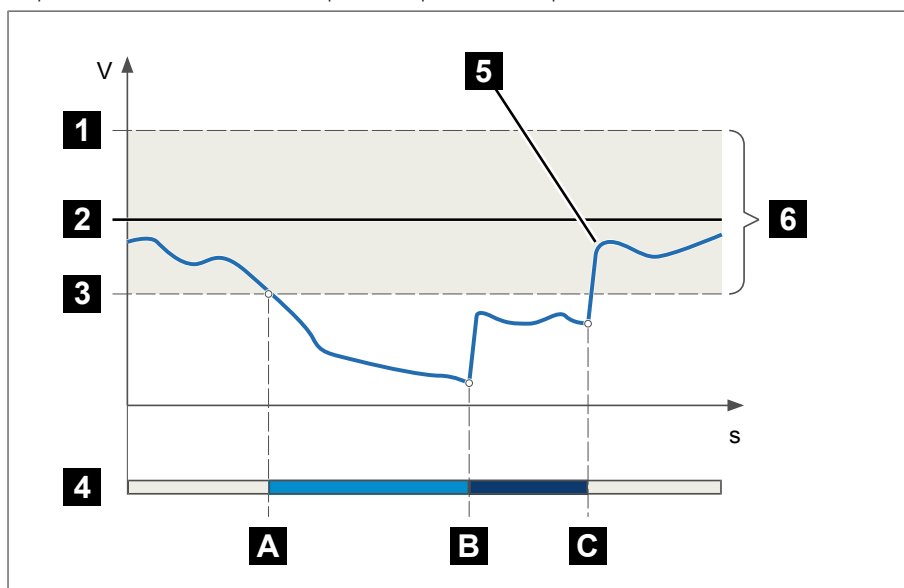
Рис. 55: Регулирование с временем задержки T1 и T2
