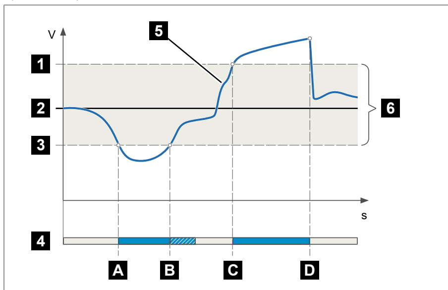
Рис. 53: Регулирование с временем задержки T1
