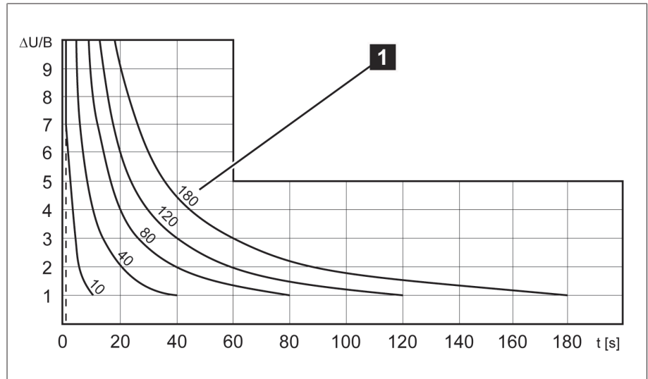
Рис. 54: Диаграмма интегрального режима времени
