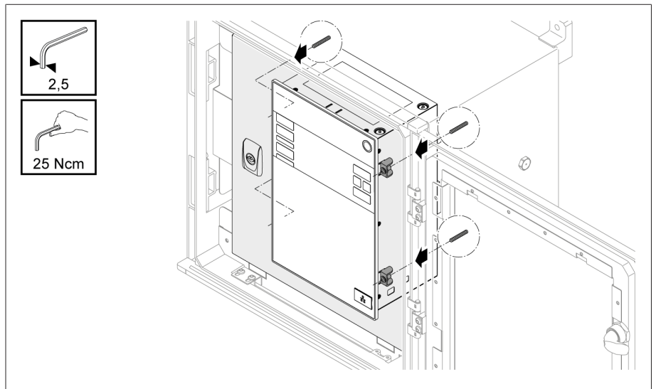
Рис. 25: Крепление устройства
