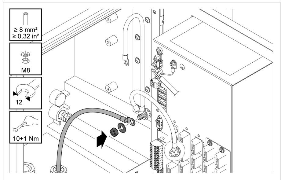
Рис. 32: Заземление корпуса
