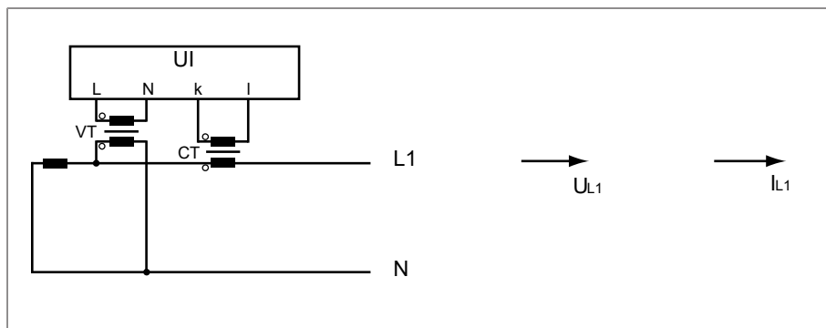
Рис. 44: Подключение 1-А
