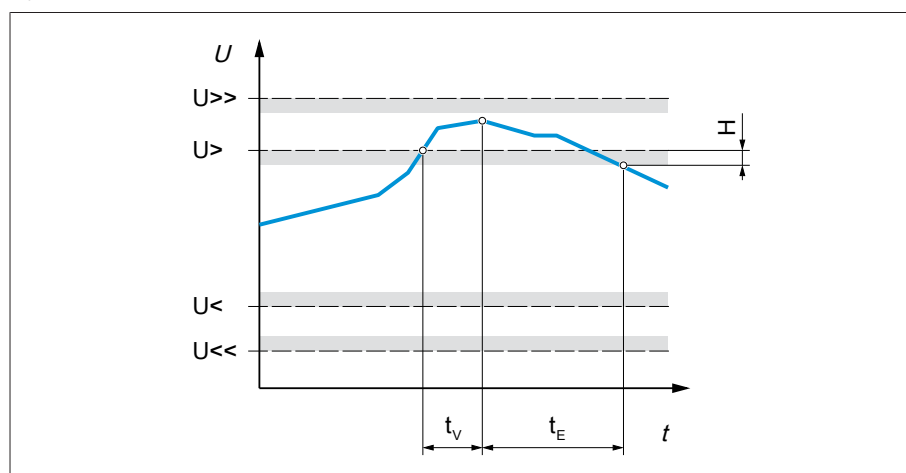
Рис. 50: Контроль напряжения с примером превышения граничного значения максимального напряжения U_{>}
