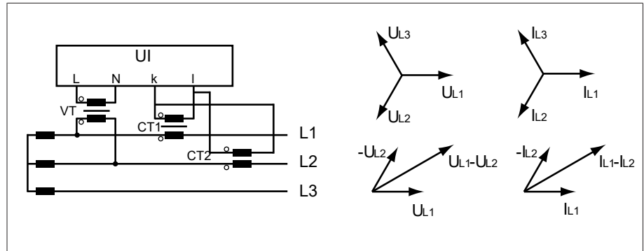
Рис. 46: Подключение 1-C
