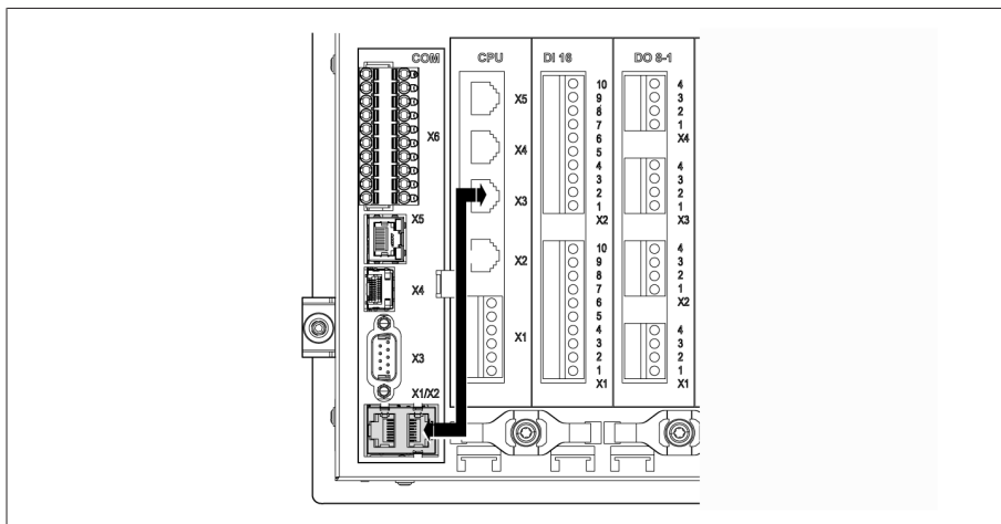
Рис. 60: Соединительный кабель с задней стороны
