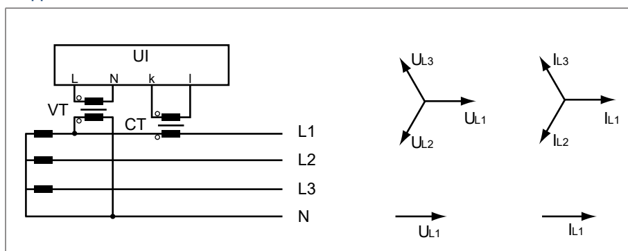
Рис. 45: Подключение 1-В
