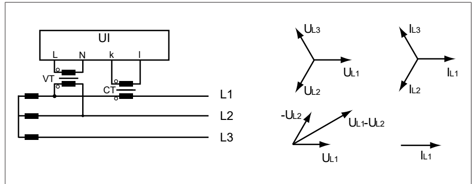
Рис. 49: Подключение 1-F
