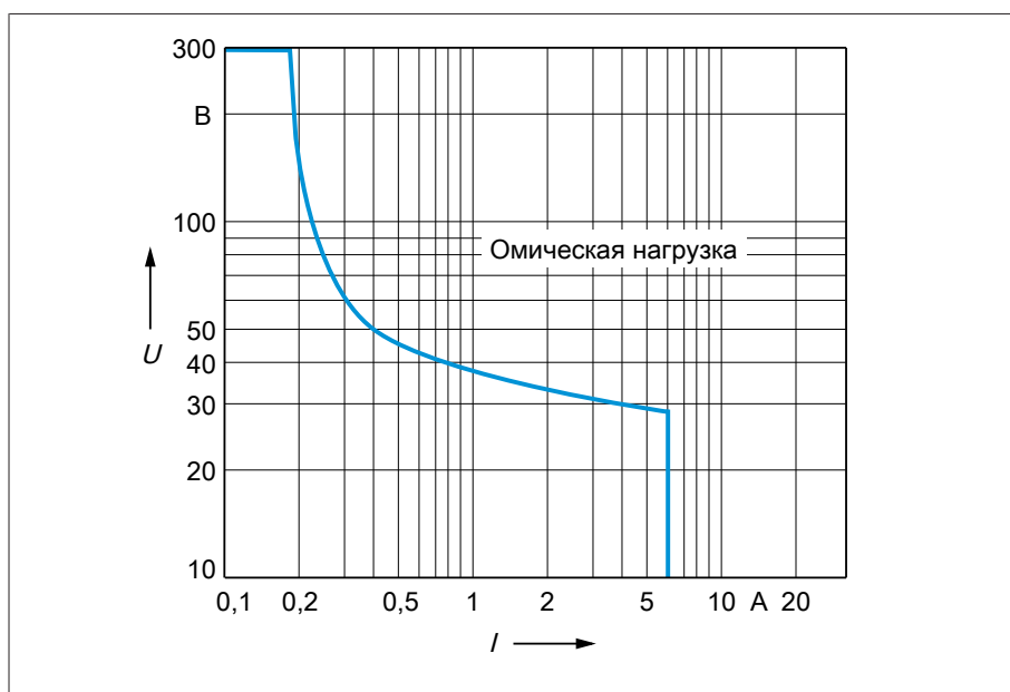
Рис. 64: Нагрузочная способность контактов цифровых выходов при активной нагрузке
