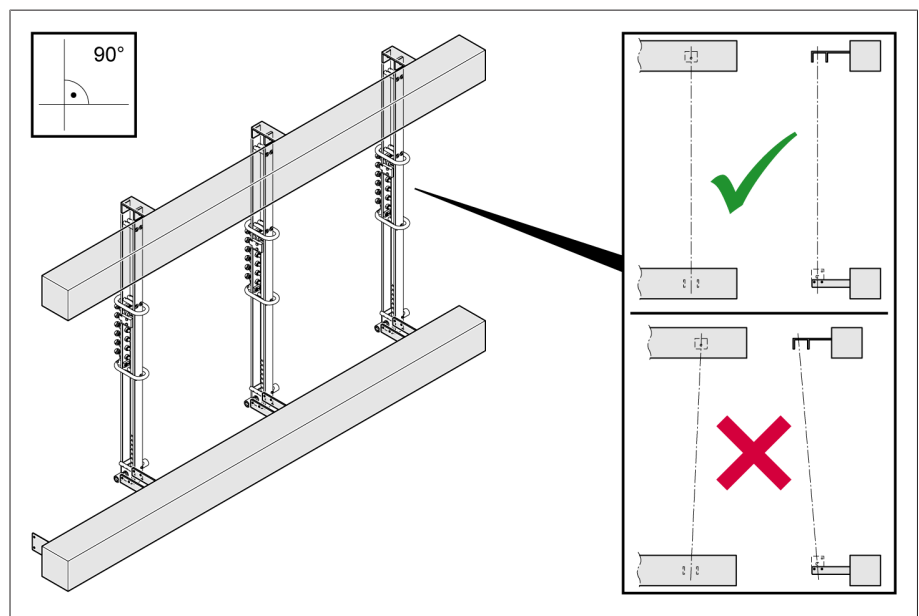
Figura 3: Dispositivos de sujeción, cambiador de tomas sin tensión con contactos colocados frontalmente
