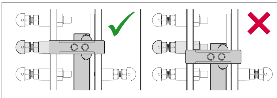
Figura 22: Contactos móviles en contacto fijo, serie de modelos MRV
