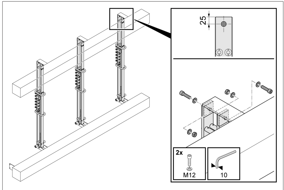
Figura 11: Fijación de la barra de soporte, cambiador de tomas sin tensión con contactos colocados frontalmente
