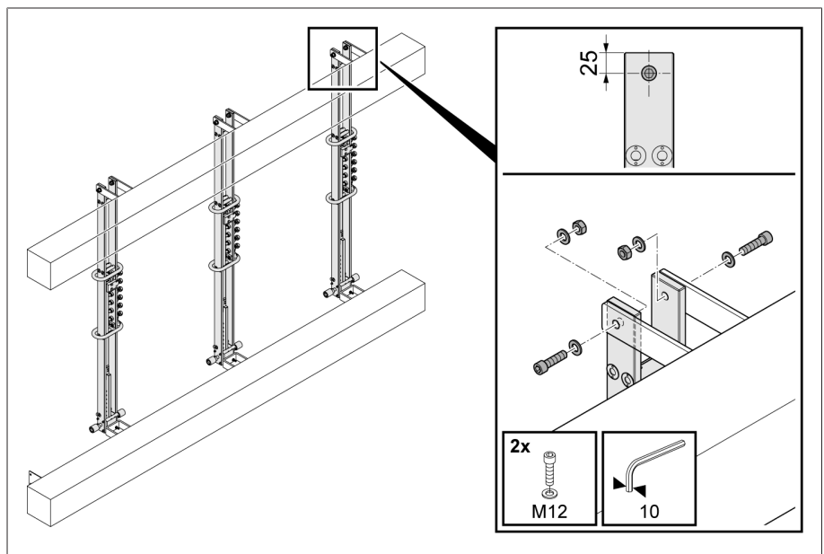
Figura 12: Fijación de la barra de soporte, cambiador de tomas sin tensión con contactos colocados lateralmente
