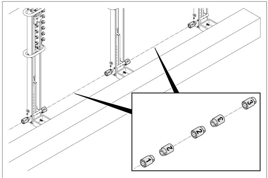
Figura 23: Árboles numerados en los engranajes reductores
