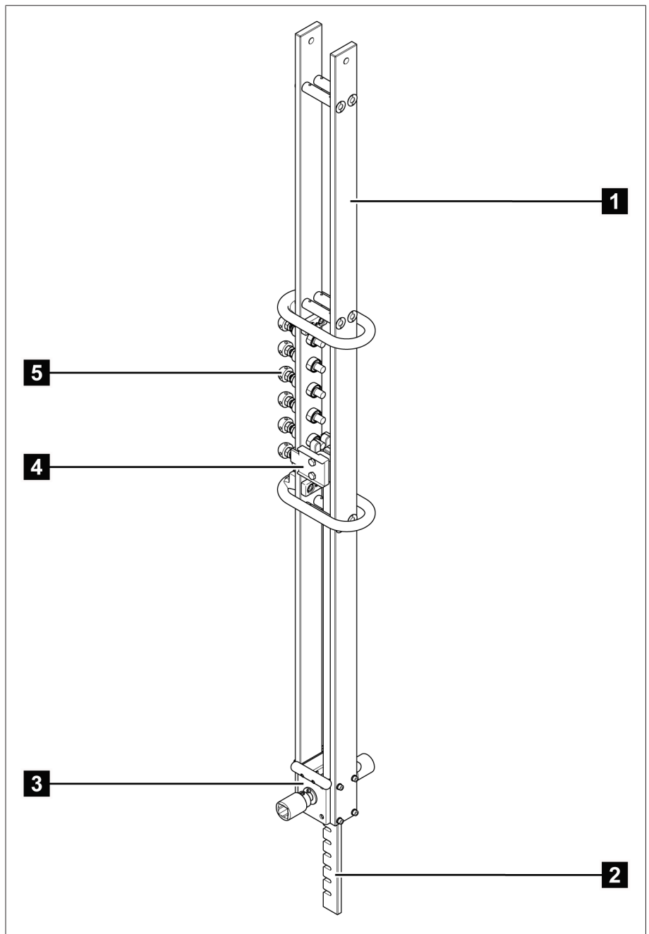
Figura 1: DEETAP® SPTM 025 con contactos colocados frontalmente
