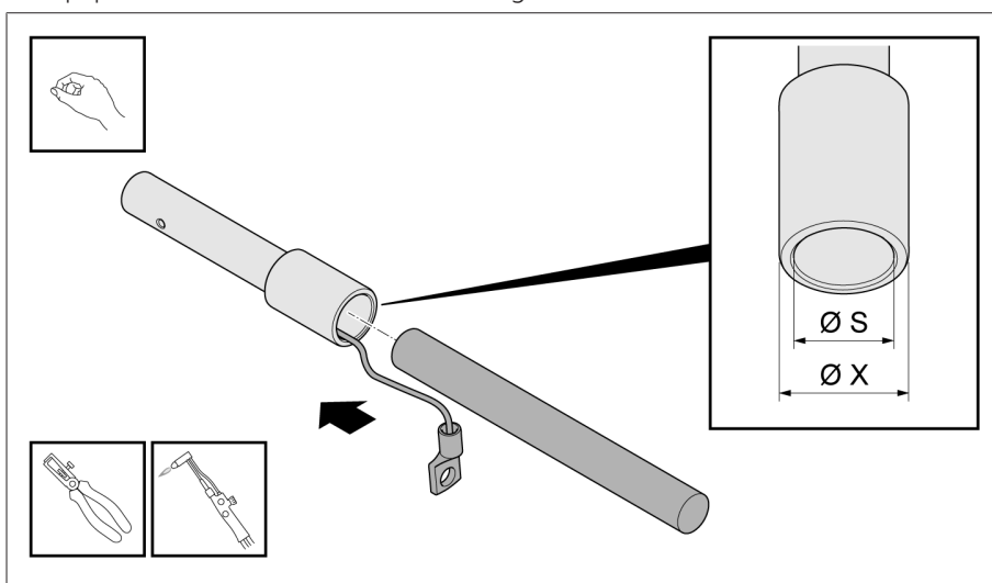
Figura 16: Fije el conductor de conexión con devanados de regulación y la conexión equipotencial en el contacto.
