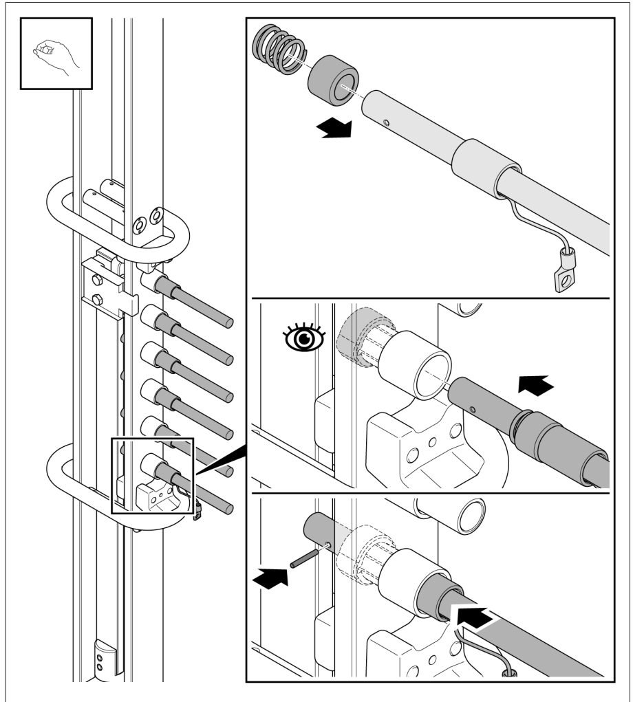
Figura 17: Fijación del contacto en el cambiador de tomas sin tensión
