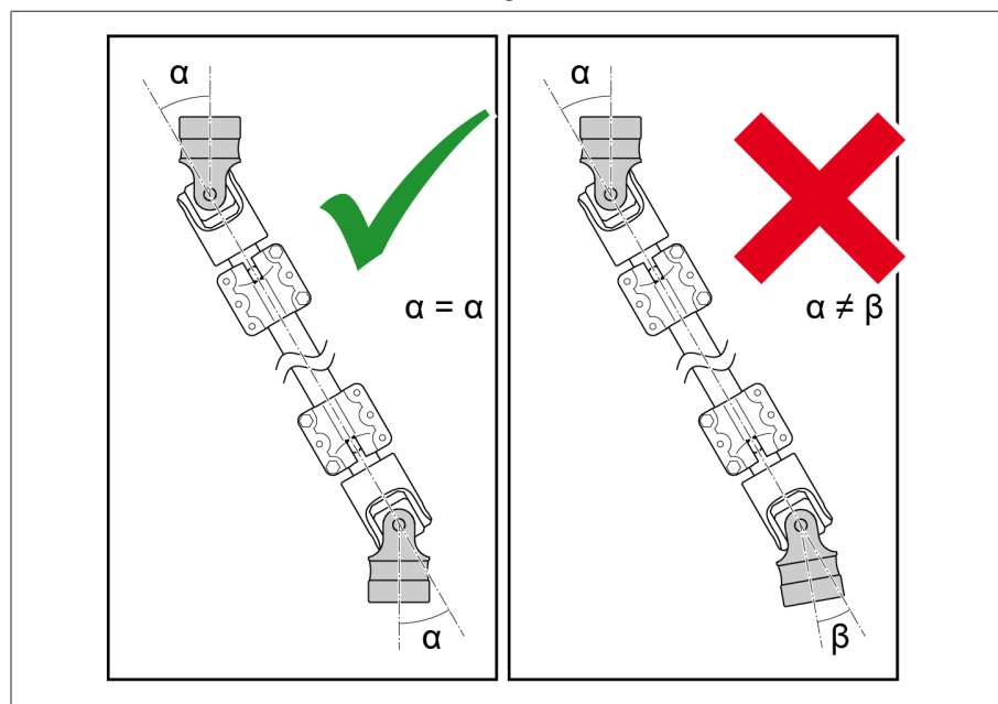
Figura 28: Ángulo de desviación \alpha
