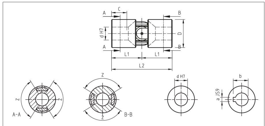
Figura 29: Zona de taladro Z
