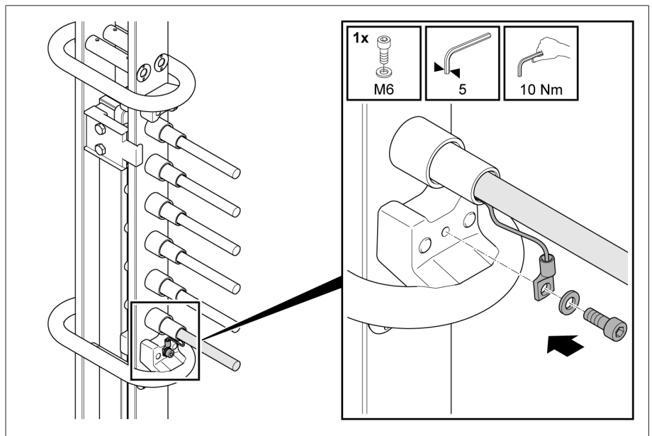
Figura 18: Fije la conexión equipotencial en el cambiador de tomas sin tensión.
