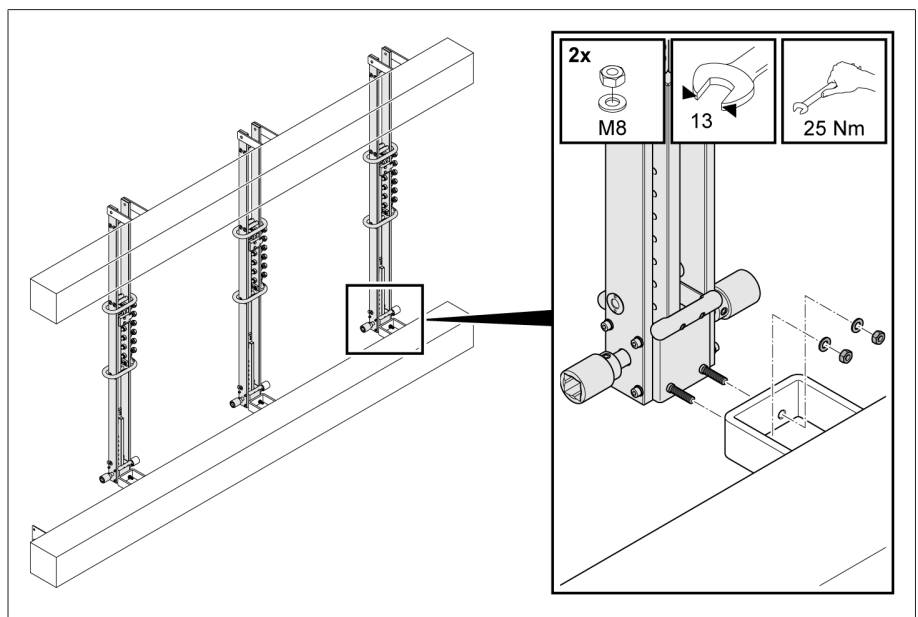
Figura 10: Fijación del engranaje reductor, cambiador de tomas sin tensión con contactos colocados lateralmente
