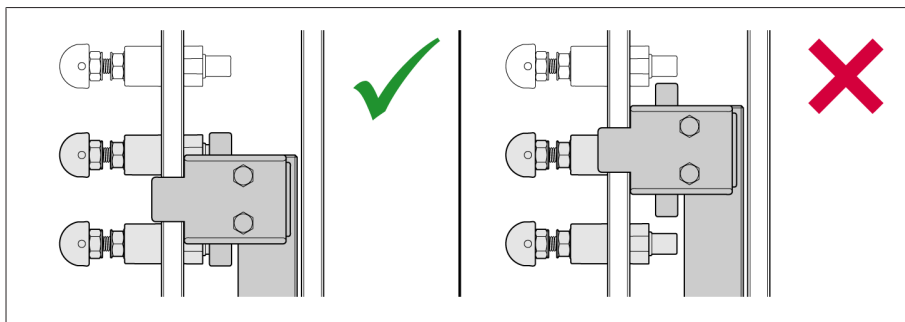
Figura 21: Contactos móviles entre 2 contactos fijos, series de modelos MTV, MTVS, MTVP, MTVD, MTVG, MTVC
