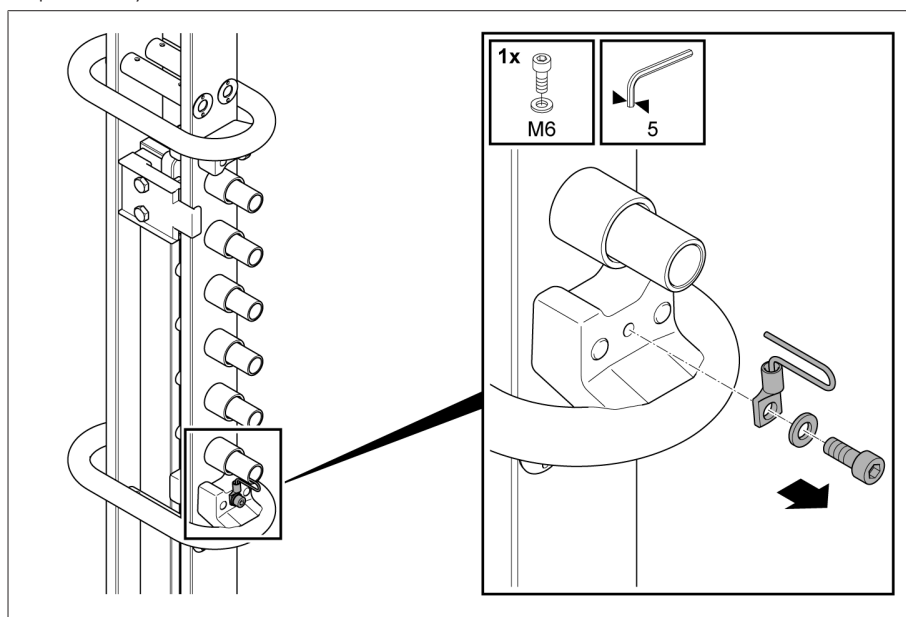
Figura 15: Eliminación de la conexión equipotencial
