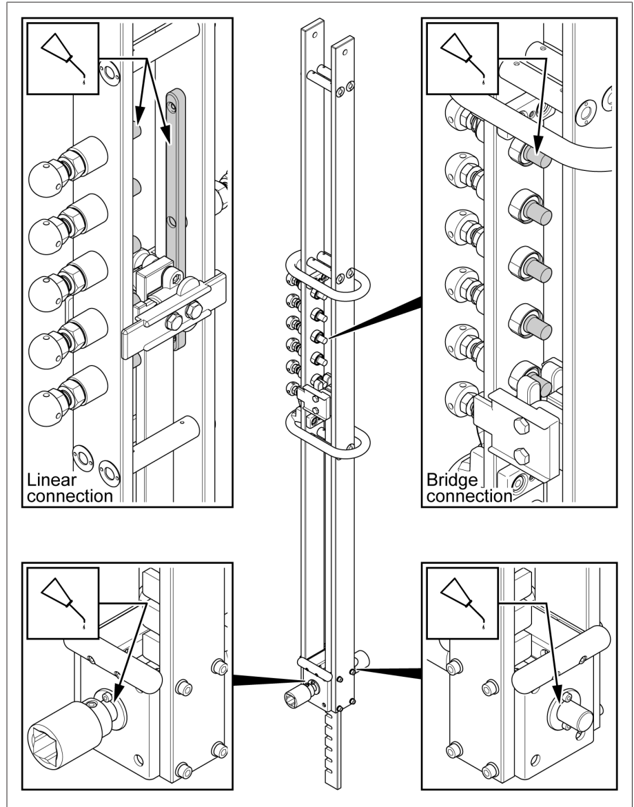
Figura 27: Puntos de lubricación
