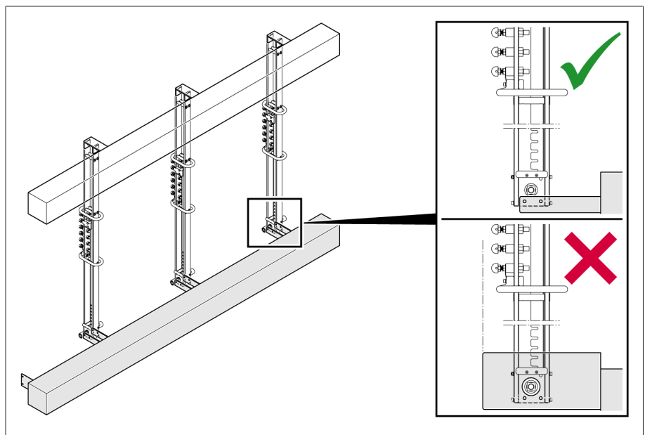
Figura 5: Dispositivo de sujeción en el engranaje reductor, cambiador de tomas sin tensión con contactos colocados frontalmente
