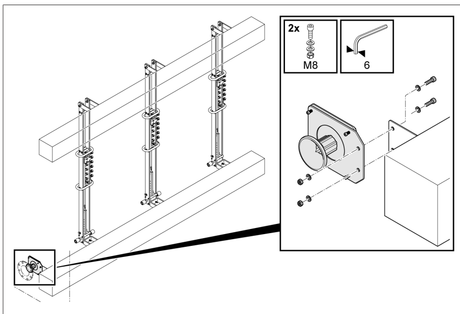
Figura 24: Acoplamiento enchufable cónico
