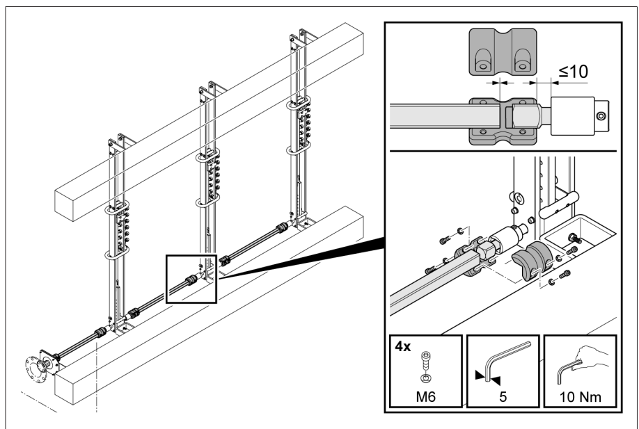
Figura 26: Casquillos de acoplamiento
