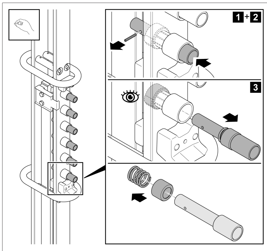
Figura 14: Extracción del contacto
