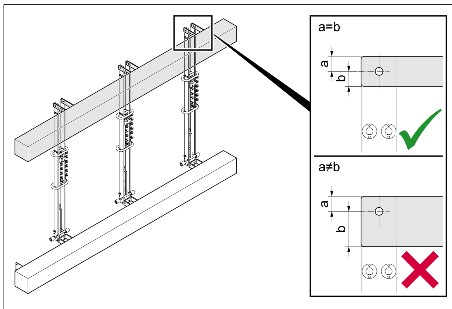
Figura 8: Dispositivo de sujeción en la barra de soporte, cambiador de tomas sin tensión con contactos colocados lateralmente
