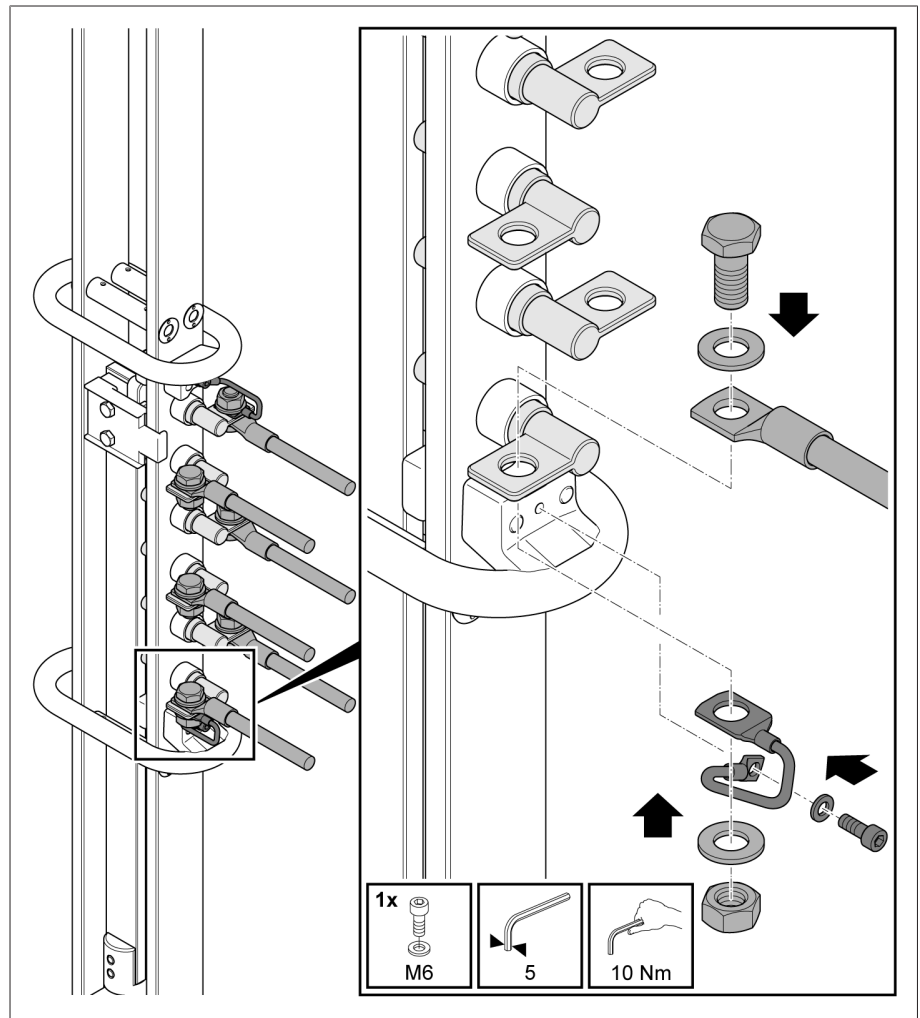
Figura 19: Conexión de conductores de conexión con devanados de regulación
