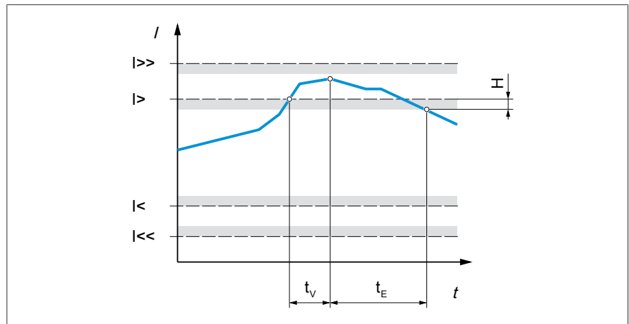
Figure 50: Surveillance du courant avec exemple de dépassement de la valeur limite I>
