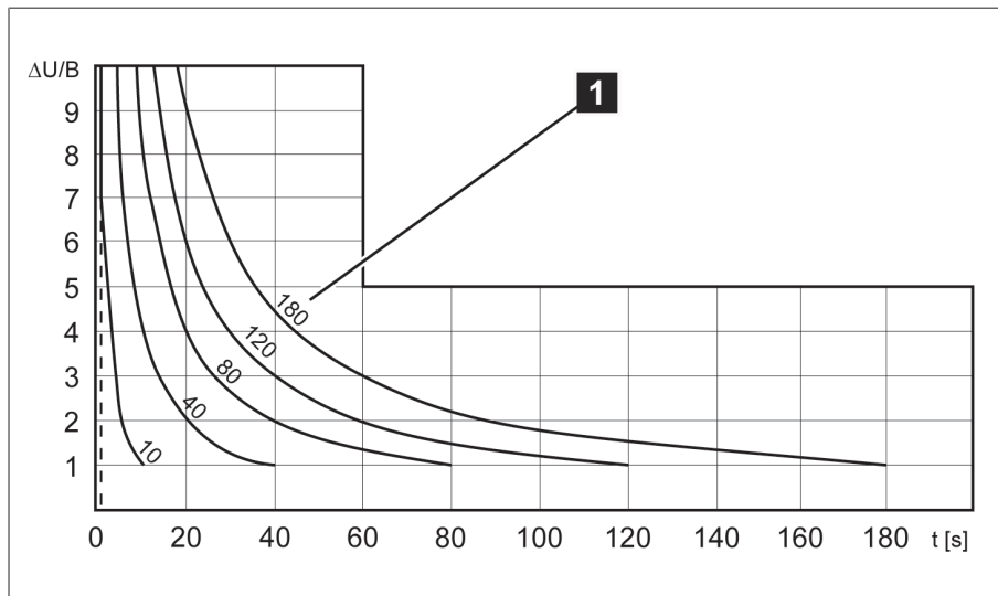
Figure 55: Diagramme de comportement temporel intégral
