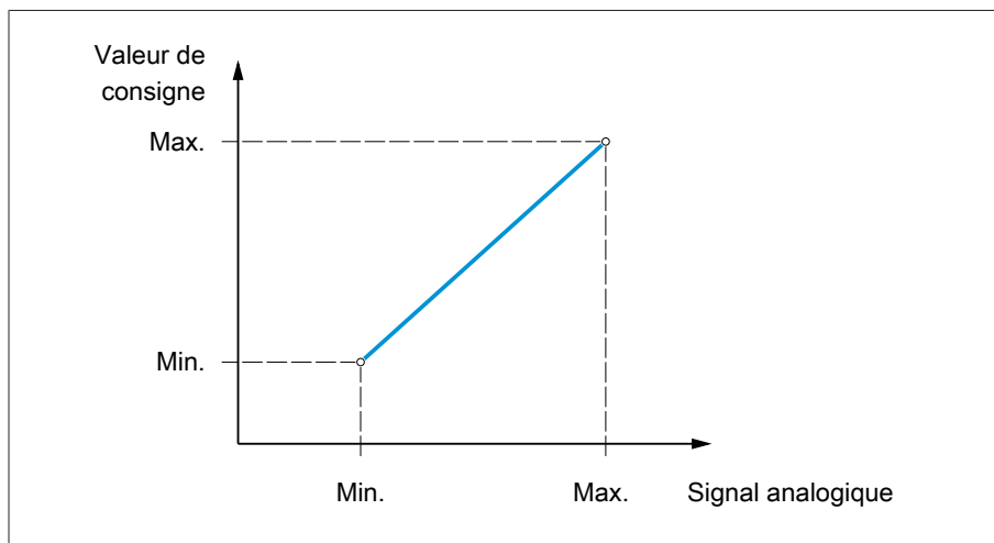
Figure 52: Valeur de consigne analogique
