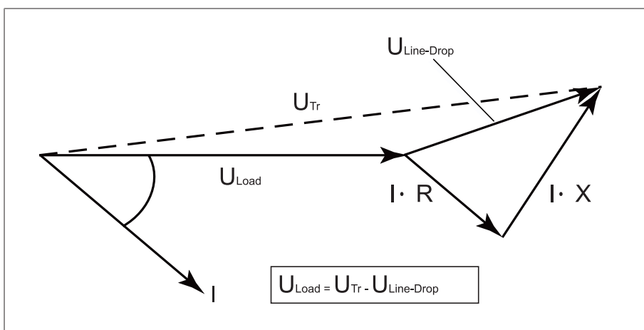
Figure 58: Représentation du curseur de la compensation R-X
