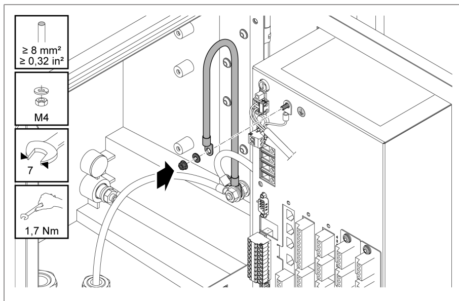
Figure 37: Fixer le câble de mise à la terre du boîtier et le conducteur de protection sur l'appareil
