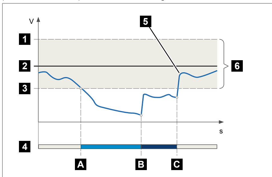
Figure 56: Comportement de la fonction de régulation avec temporisation T1 et T2
