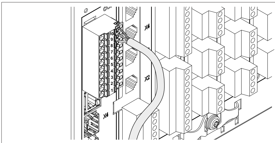
Figure 28: Raccorder les fils aux broches 10 ; 9 ; 8
