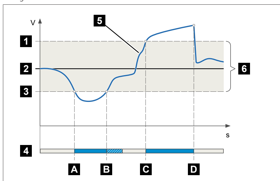
Figure 54: Comportement de la fonction de régulation avec temporisation T1
