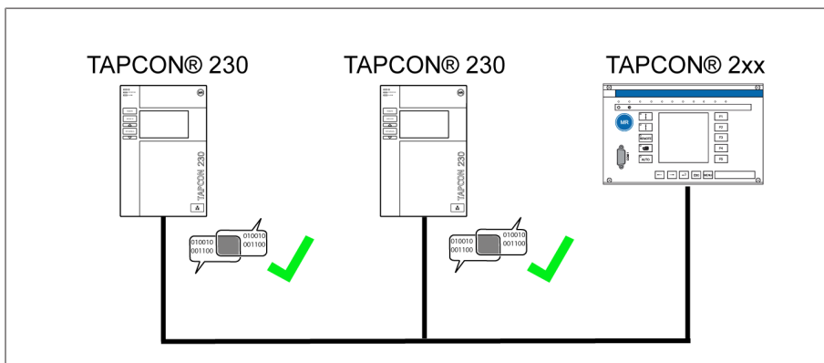
Figure 51: Marche en parallèle de 2 appareils avec un TAPCON® 2xx
