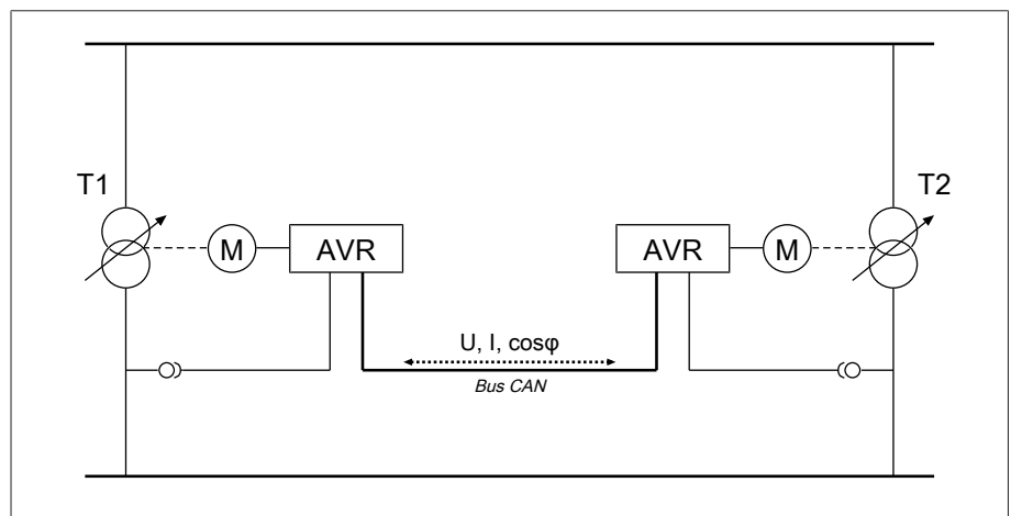
Figure 61: Minimisation du courant réactif de circulation avec communication via le bus CAN
