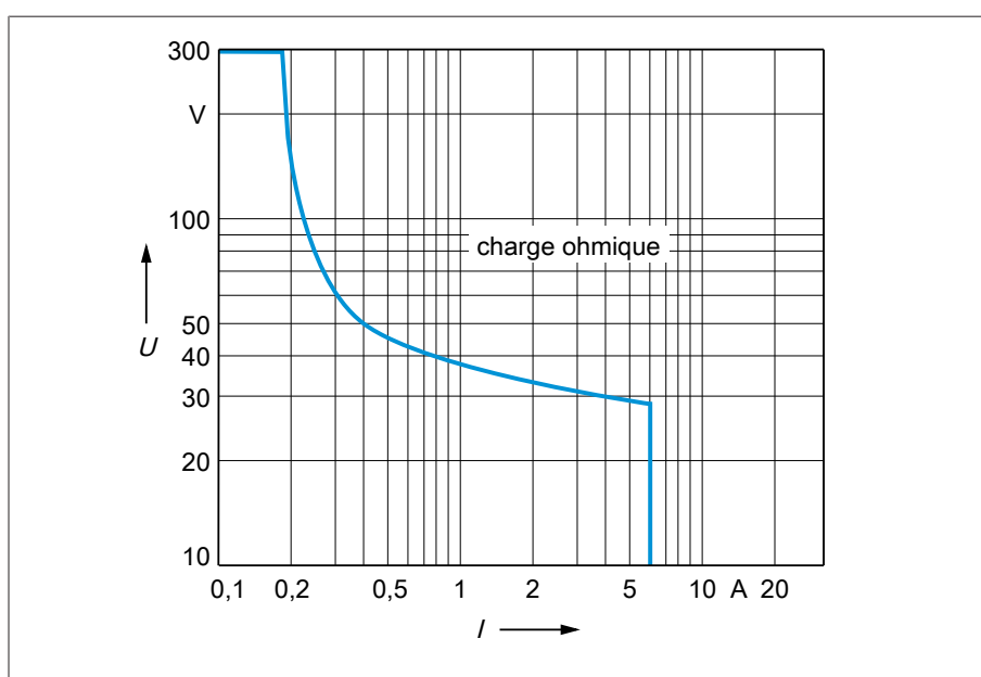
Figure 66: Capacité de charge des sorties numériques en cas de charge ohmique
