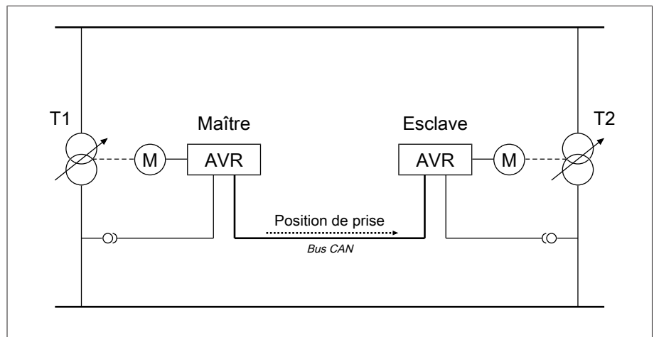
Figure 60: Synchronisation de prise
