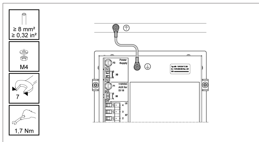
Figure 35: Raccordement du câble de terre
