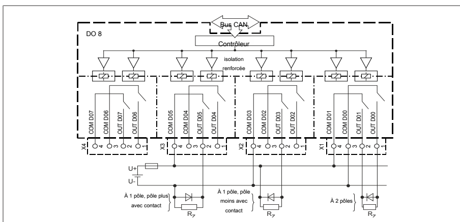
Figure 34: Schéma bloc pour les sorties numériques
