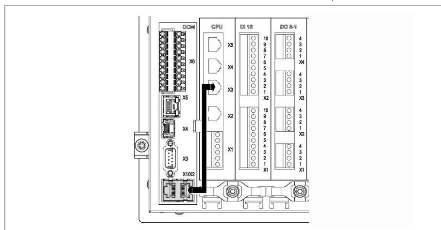
Figure 64: Câble patch sur la face arrière
