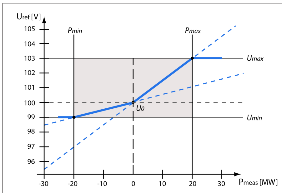
Figure 53: Adaptation de la valeur de consigne de tension en fonction de la puissance active
