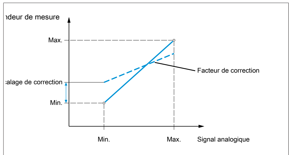
Figure 41: Signal analogique avec courbe caractéristique linéaire, facteur de correction <1 et décalage de correction
