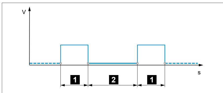
Figure 63: Durée de l'impulsion de manœuvre et pause de l'impulsion de manœuvre
