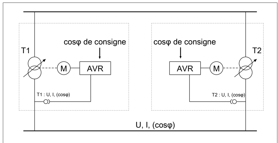
Figure 62: Minimisation du courant réactif de circulation sans communication via le bus CAN
