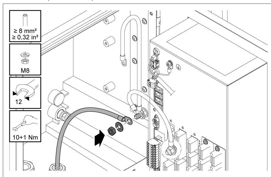
Figure 36: Mettre le boîtier à la terre
