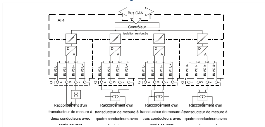
Figure 33: Schéma bloc pour les entrées analogiques
