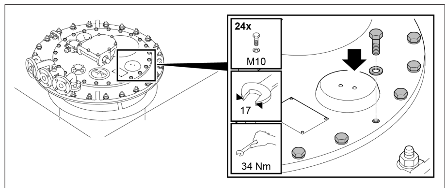
그림 192: 부하시 탭 절환장치 헤드 커버
