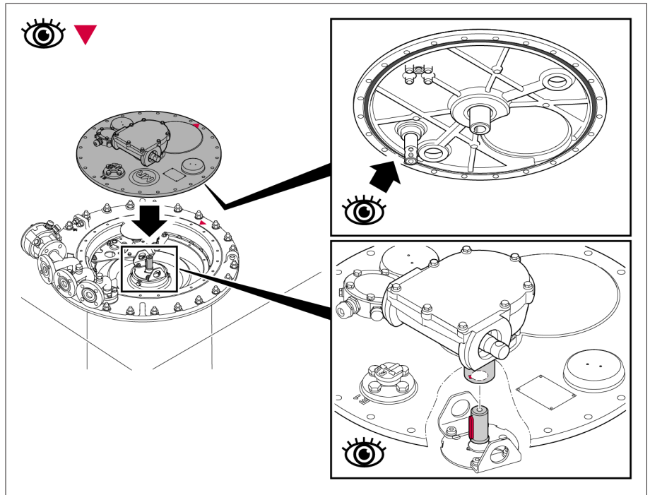
그림 59: O-링이 있는 부하시 탭 절환장치 헤드 커버
