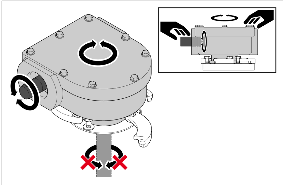
그림 257: 기어 유닛 정렬하기
