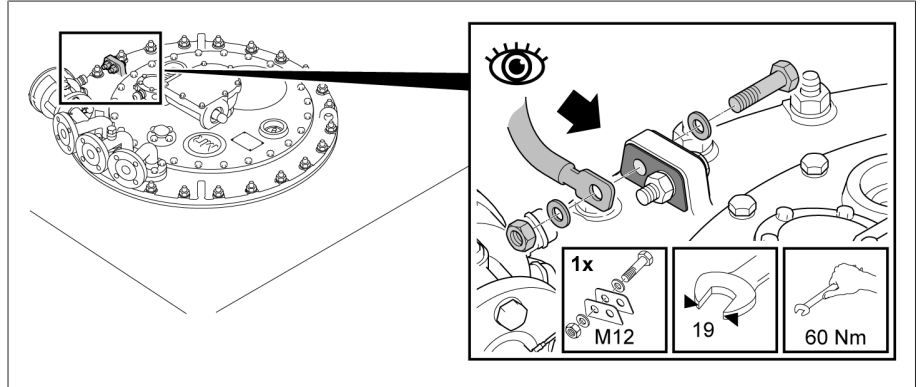
그림 316: 접지 나사 헤드
