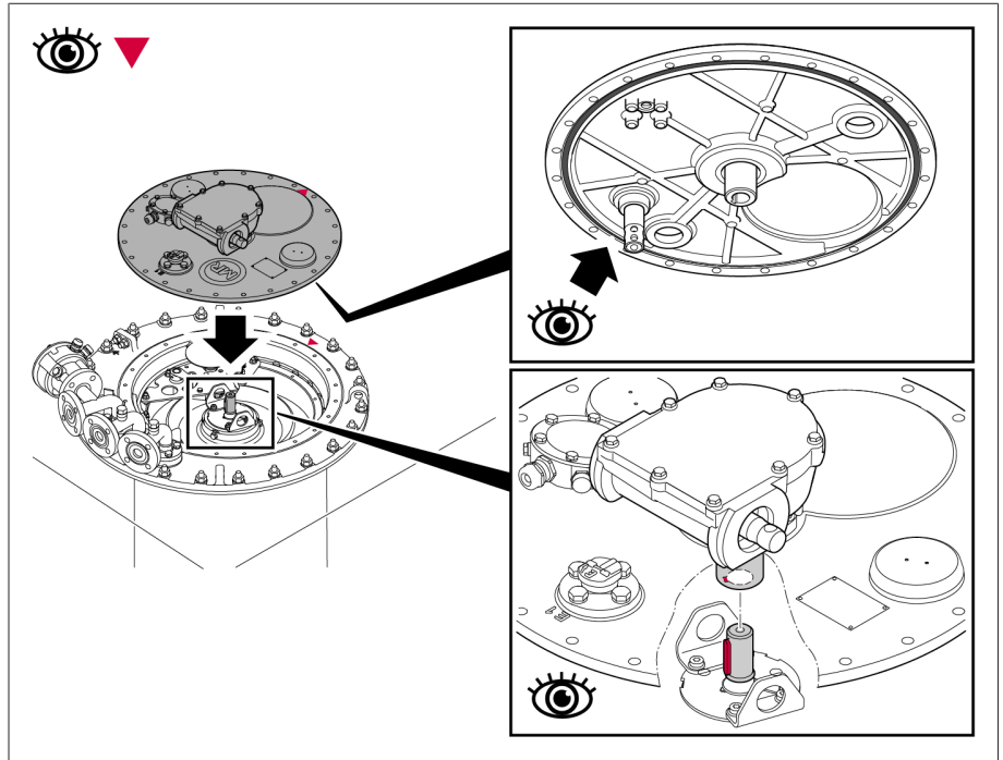
그림 115: O-링이 있는 부하시 탭 절환장치 헤드 커버
