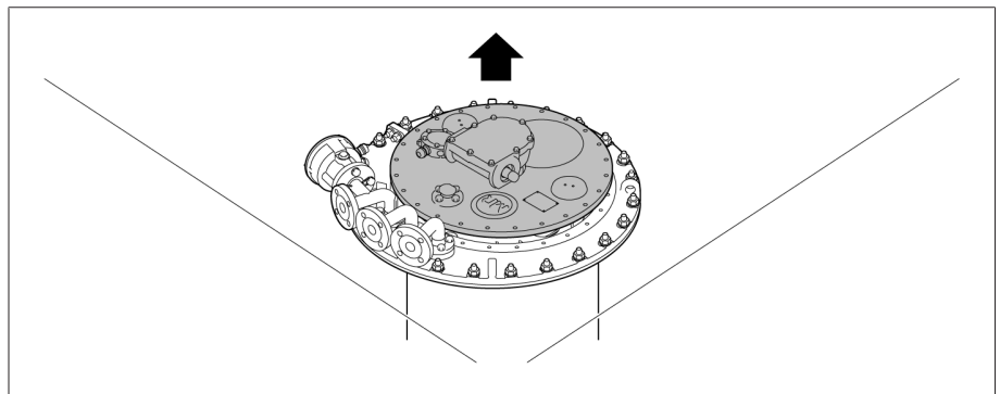
그림 195: 부하시 탭 절환장치 헤드 커버
