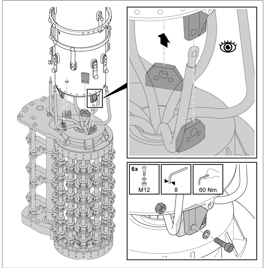
그림 70: 선택기를 유격실에 나사로 고정하기
