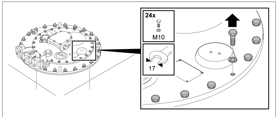
그림 194: 부하시 탭 절환장치 헤드 커버
