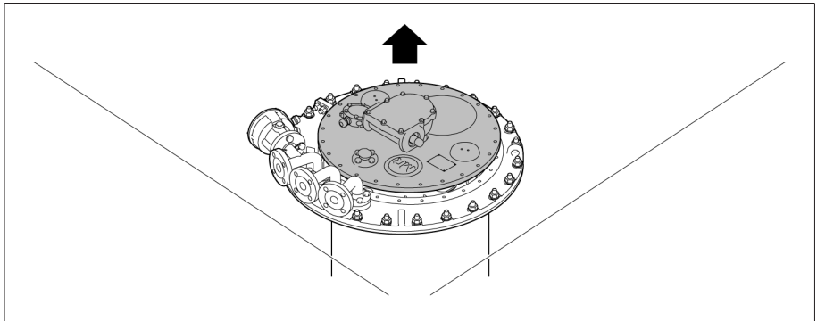
그림 150: 부하시 탭 절환장치 헤드 커버
