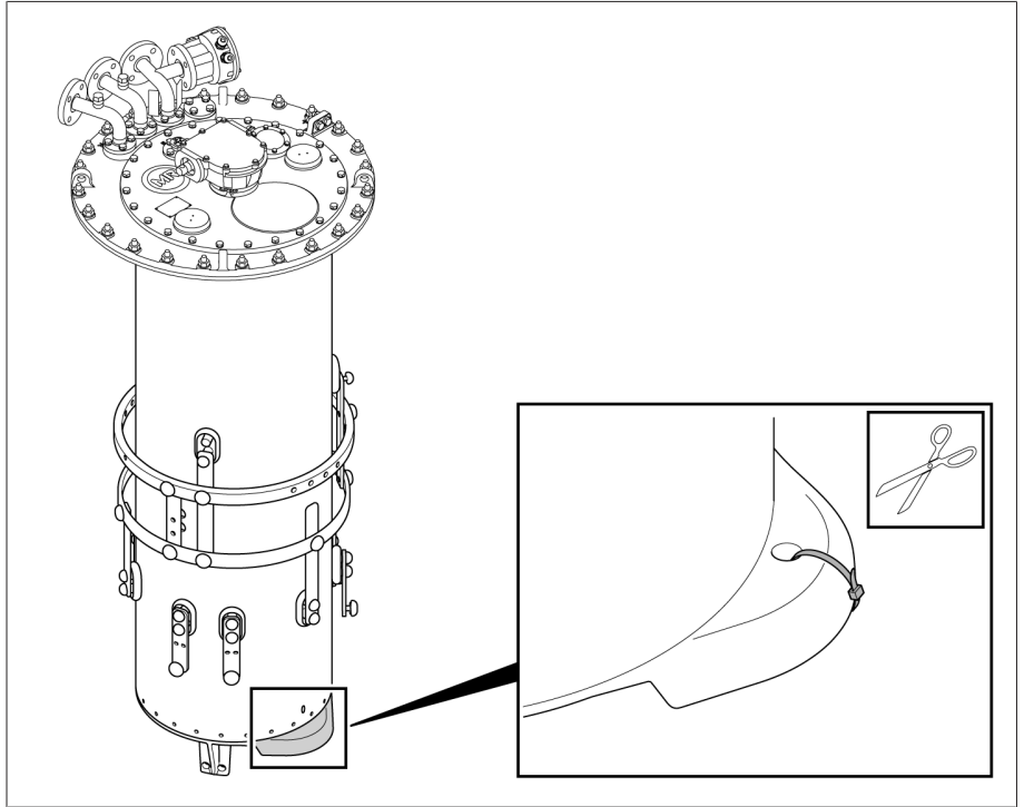
그림 46: 잠금 밴드가 있는 유격실 하부
