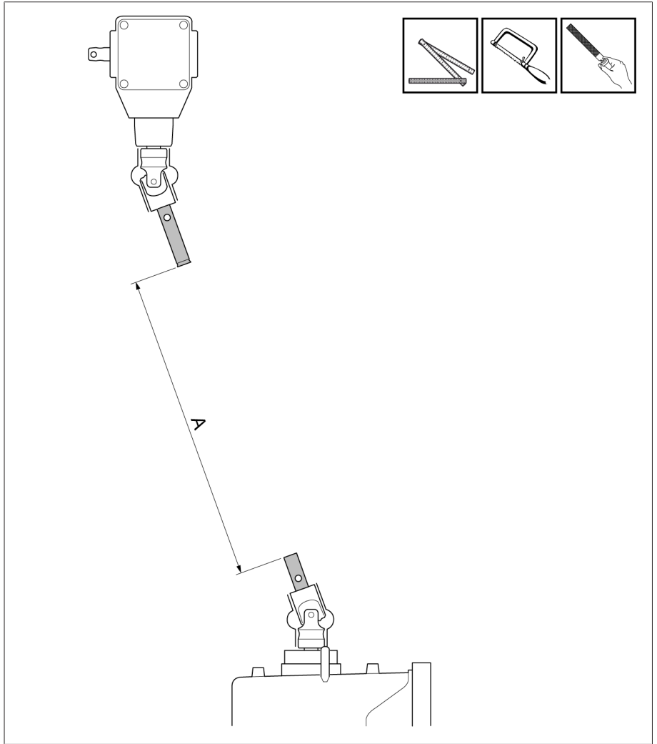
그림 286: 신축 튜브 줄이기
