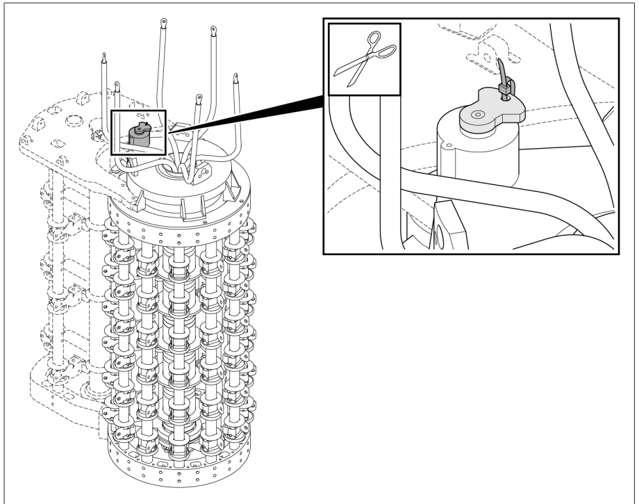
그림 127: 잠금 밴드가 있는 탭 선택기 커플링
