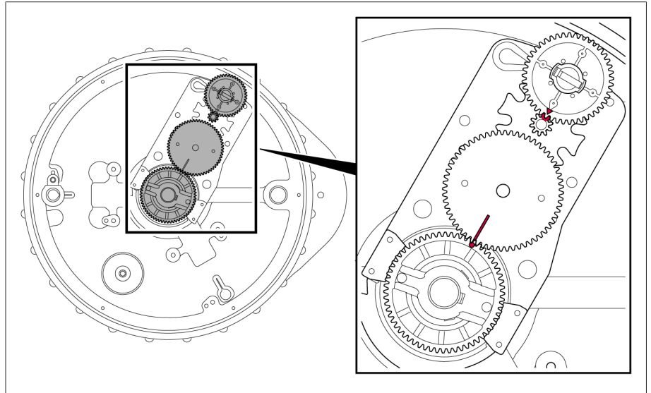
그림 204: 유격실 하부에 있는 조정 표시
