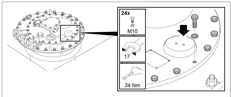
그림 148: 부하시 탭 절환장치 헤드 커버
