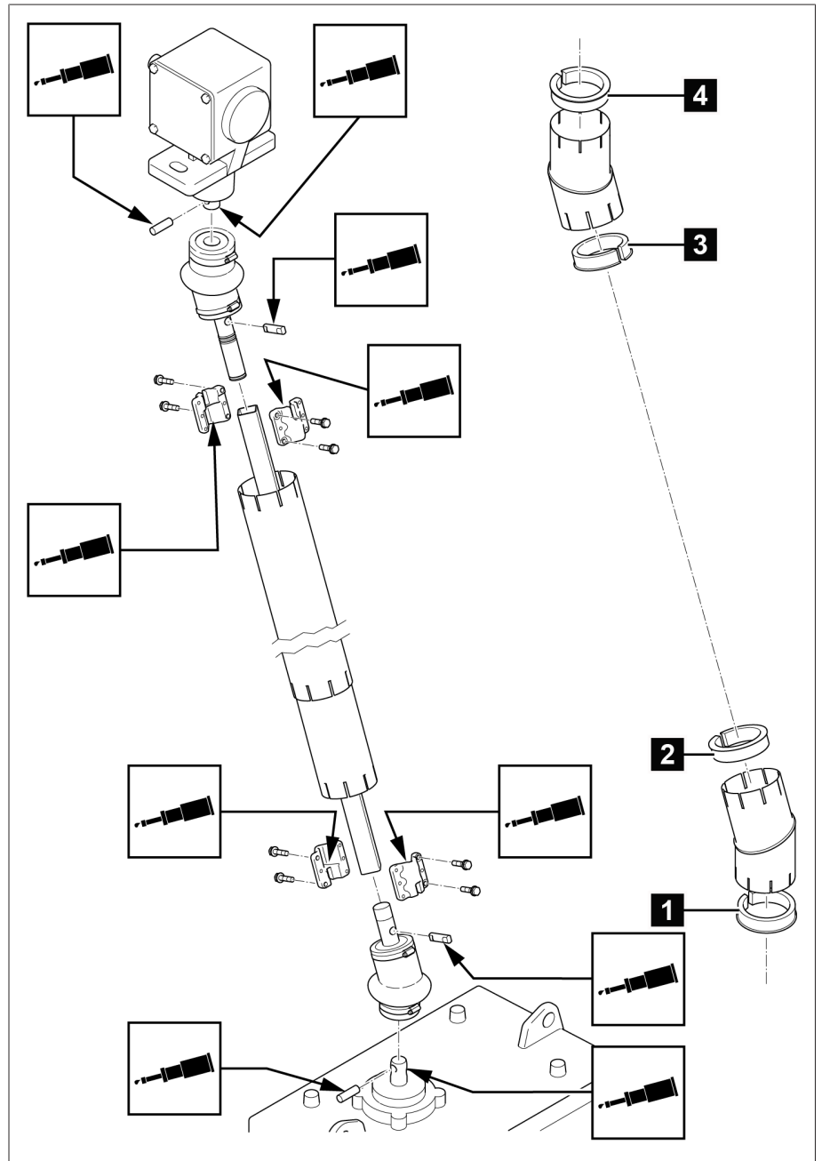
그림 278: 연결 볼트, 연결 브래킷 및 중공축에 그리스 바르기
