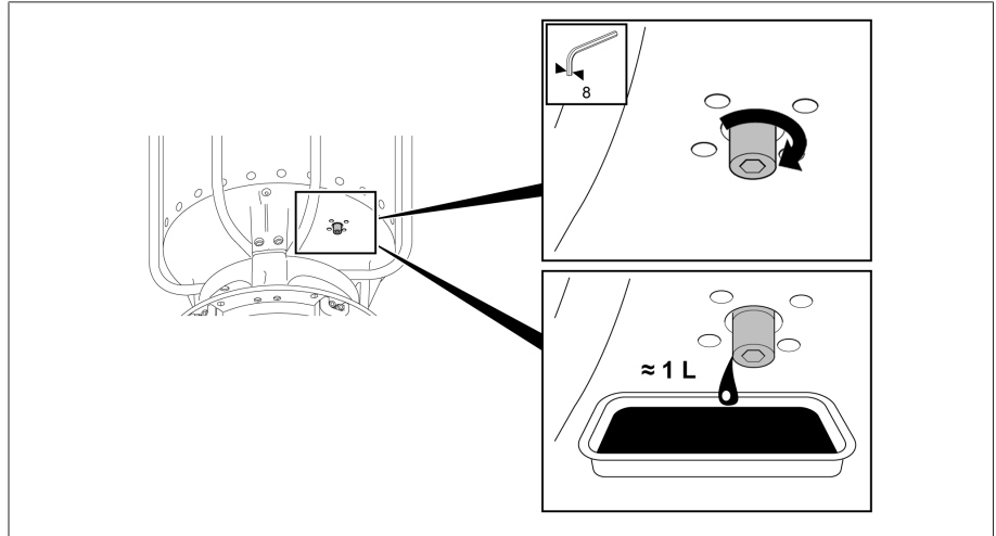
그림 89: 등유 배출 플러그
