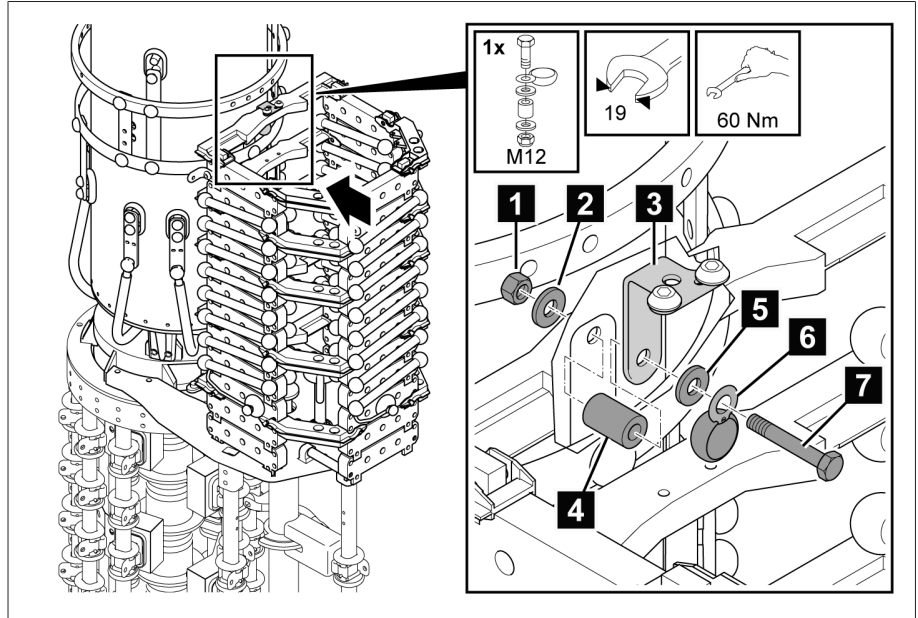
그림 134: 전위연결 기구 고정
