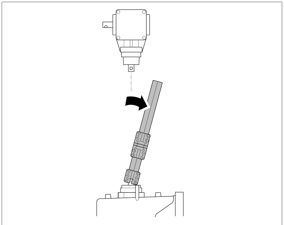
그림 306: 사각 관을 돌려 축에서 떨어뜨리기
