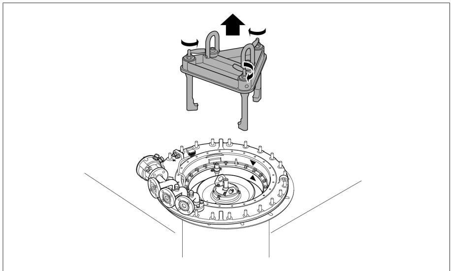
그림 177: 리프팅 장비 제거하기
