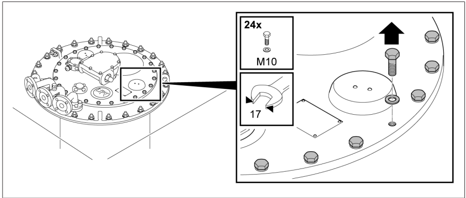
그림 149: 부하시 탭 절환장치 헤드 커버
