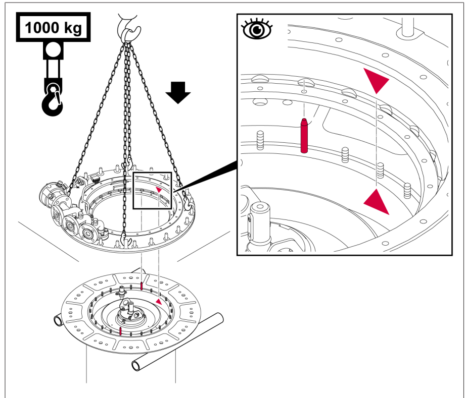
그림 173: 표시와 정렬 핀
