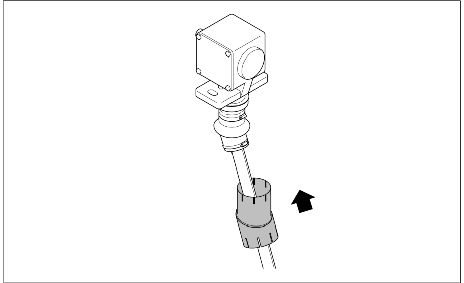
그림 289: 회전 가능 보호 튜브를 사각 관 위에 끼우기
