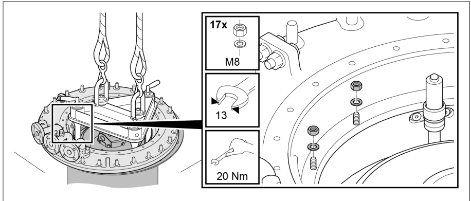
그림 176: 부하시 탭 절환장치 헤드의 상단을 하단에 나사로 고정하기
