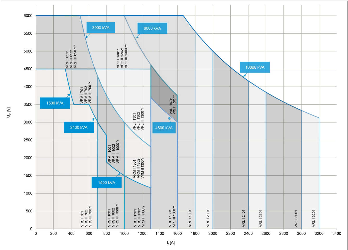
그림 326: 스텝 용량(정격 전압 U_r , 정격 통과 전류 I_r ), *로 표시된 부하시 탭 절환장치 유형은 특수한 응용 모델이며, 요청 시에만 사용할 수 있습니다.
