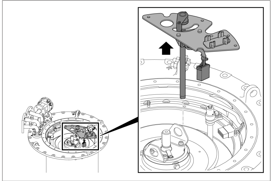
그림 99: 탭 변환 감시 장치 및 구동축과 마운팅 플레이트
