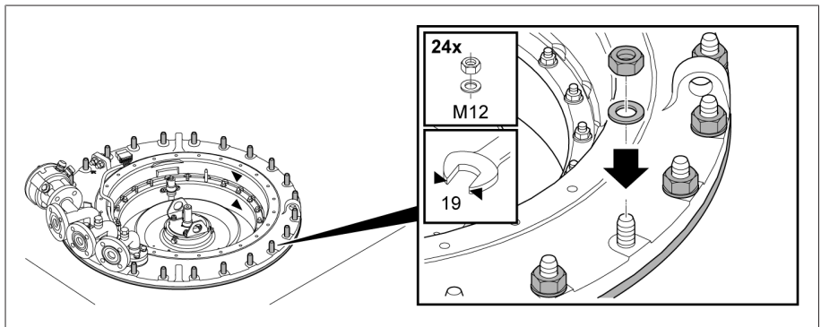
그림 178: 부하시 탭 절환장치 헤드를 마운팅 플랜지에 나사로 고정하기
