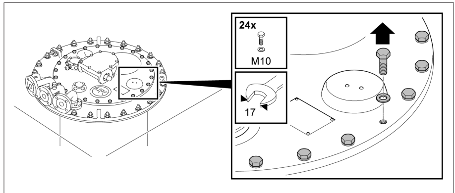
그림 87: 부하시 탭 절환장치 헤드 커버
