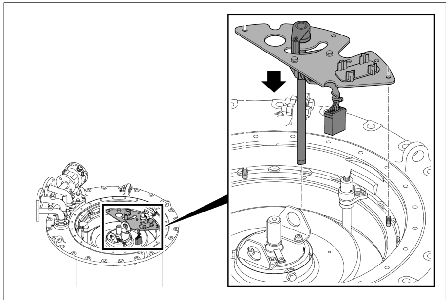
그림 182: 탭 변환 감시 장치 및 구동축과 마운팅 플레이트
