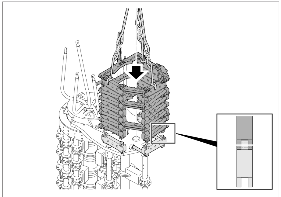
그림 62: 전위연결 기구 내리기
