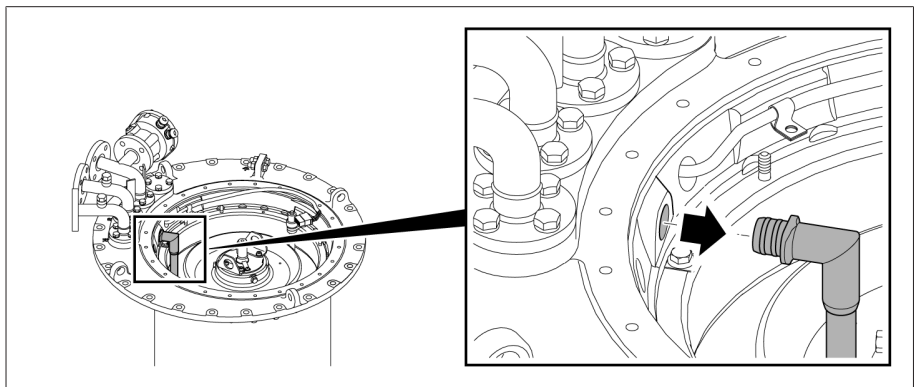
그림 166: 오일 흡입 파이프
