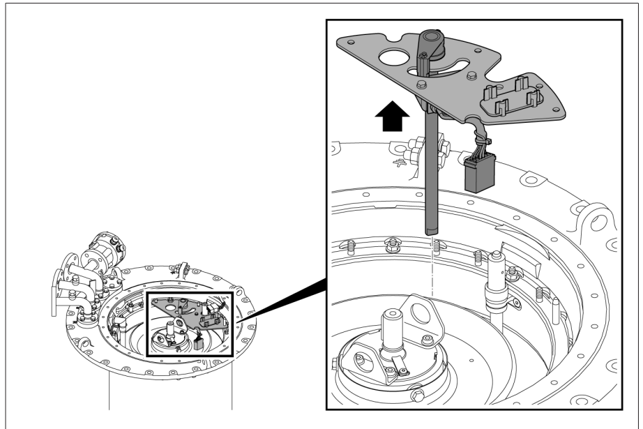
그림 161: 탭 변환 감시 장치 및 구동축과 마운팅 플레이트
