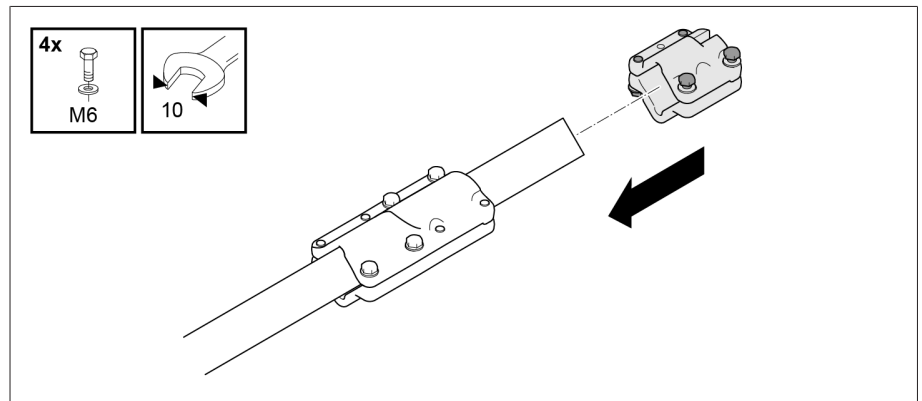
그림 302: 연결 부품을 밀어서 절연체에 끼우기
