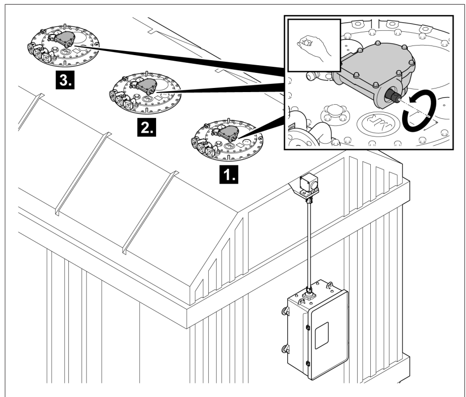
그림 271: 부하시 탭 절환장치 컬럼 수동으로 전환하기
