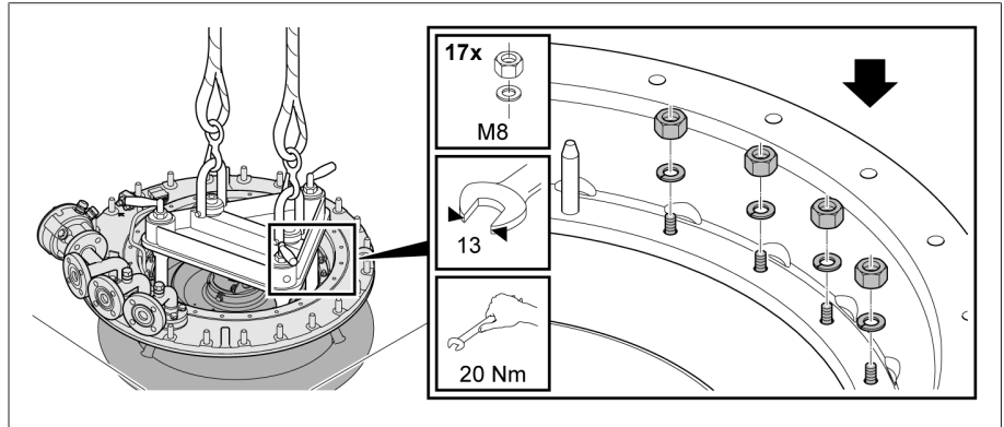
그림 43: 부하시 탭 절환장치 헤드 상단을 하단에 나사로 고정하기
