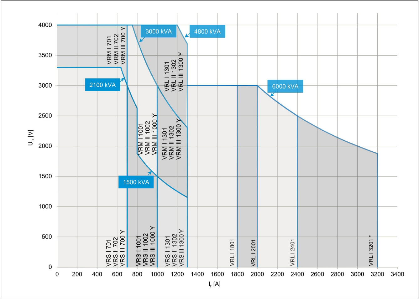
그림 327: 스텝 용량(정격 전압 U_s , 정격 통과 전류 I_s ), *로 표시된 부하시 탭 절환장치 유형은 요청 시에만 사용할 수 있습니다.
