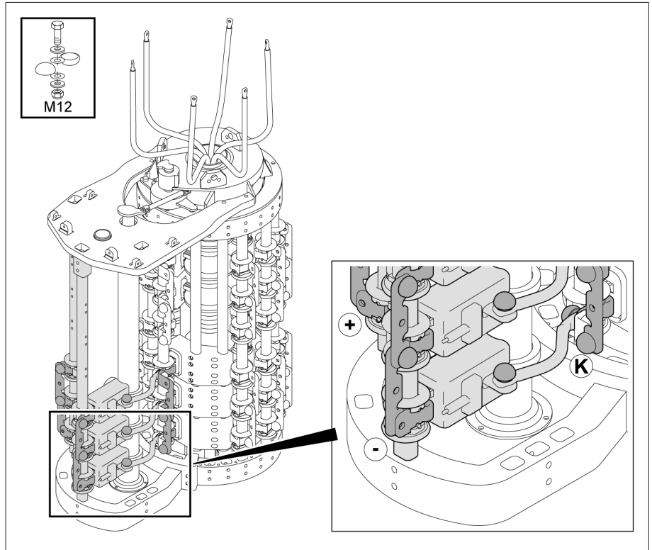
그림 78: 리버싱 체인지 오버 선택기 결선용 체인지 오버 선택기 연결 접점
