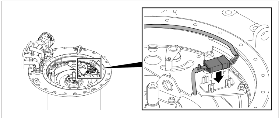
그림 212: 브래킷에 끼운 플러그 커넥터
