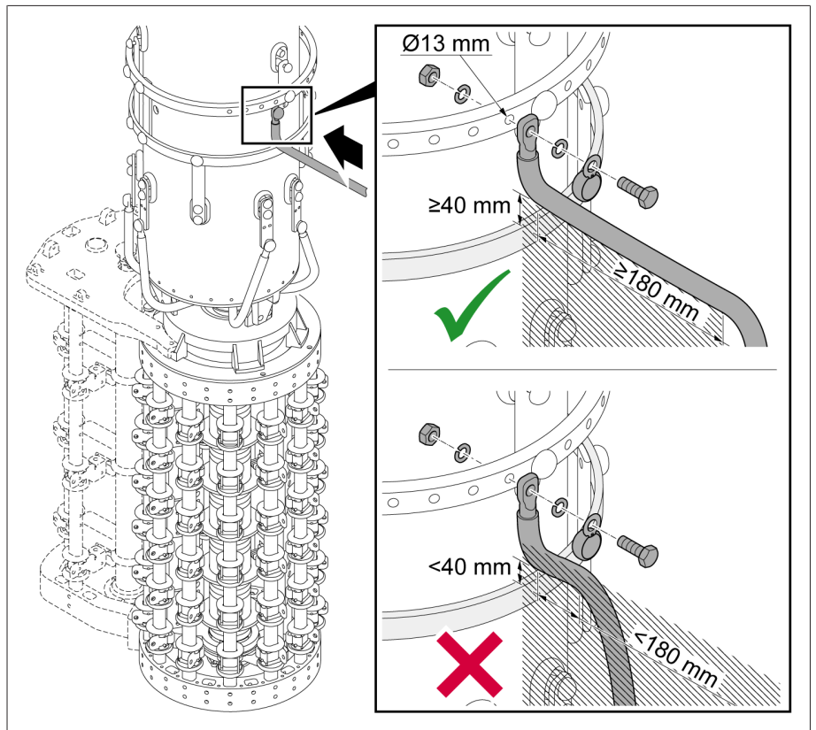
그림 81: 유격실의 인출 링
