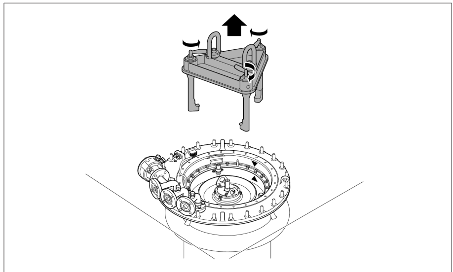
그림 44: 리프팅 장비 제거하기
