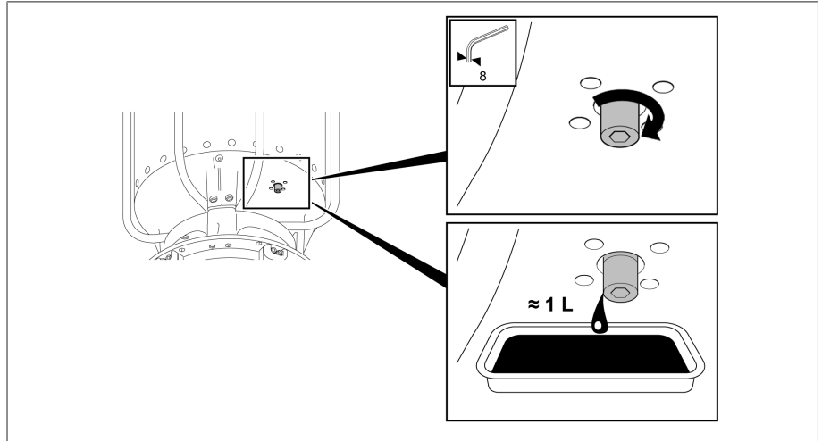
그림 151: 등유 배출 플러그
