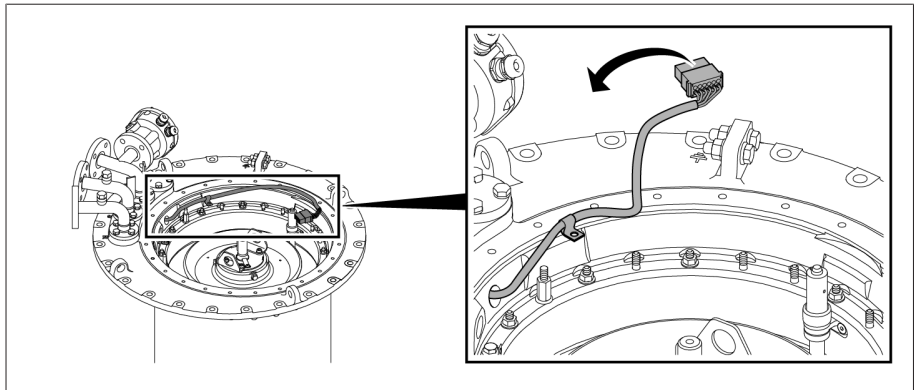
그림 31: 탭 변환 감시 장치의 케이블
