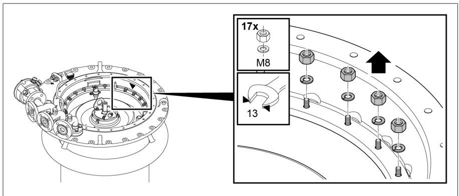
그림 36: 부하시 탭 절환장치 헤드의 상단과 하단을 결합하는 너트와 잠금 소자
