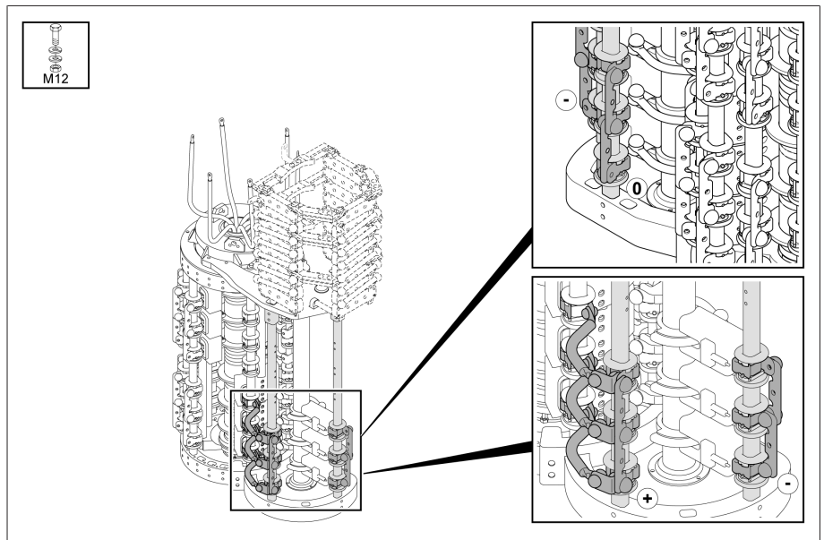
그림 141: 코스 탭 선택기 결선용 체인지 오버 선택기 연결 접점
