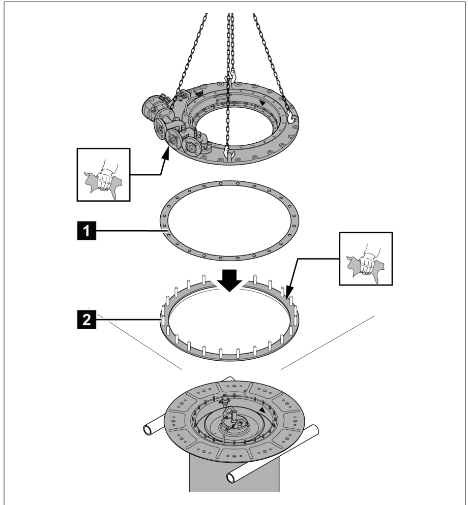
그림 172: 개스킷이 있는 마운팅 플랜지
