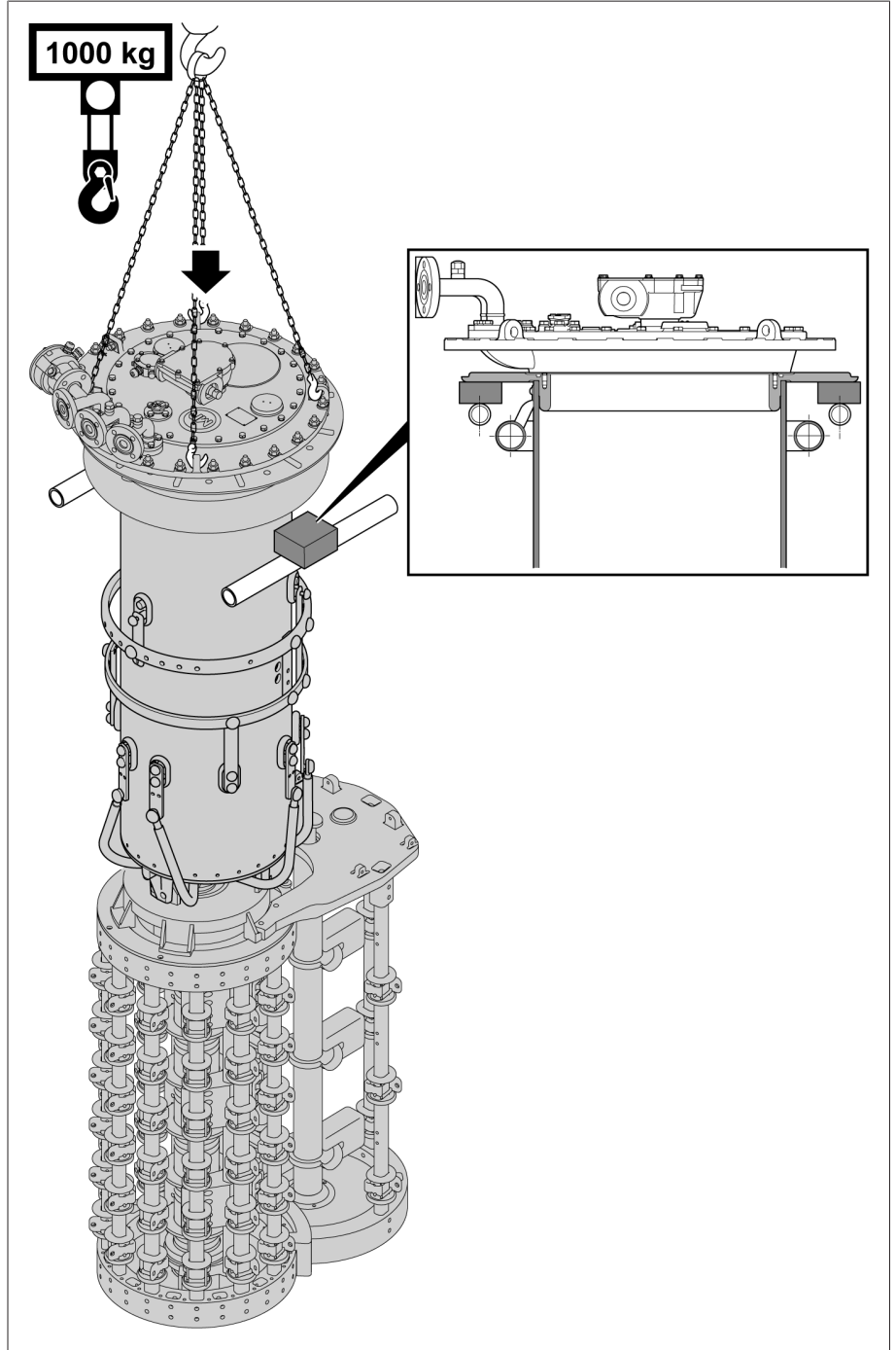
그림 135: 부하 지지 구조물 위에 스페이서가 있는 부하시 탭 절환장치
