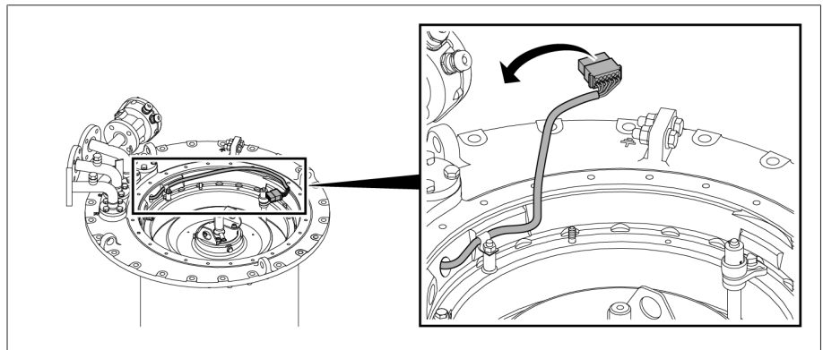
그림 200: 탭 변환 감시 장치의 케이블
