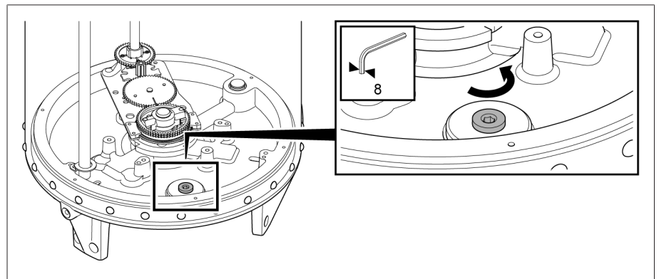
그림 203: 등유 배출 플러그
