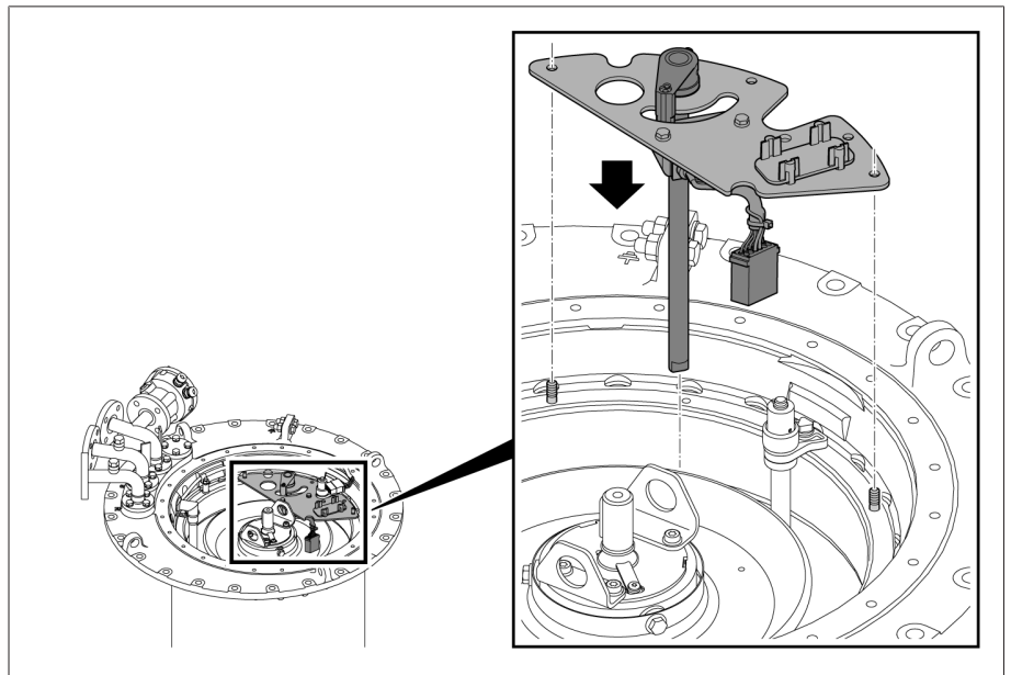
그림 50: 탭 변환 감시 장치 및 구동축과 마운팅 플레이트
