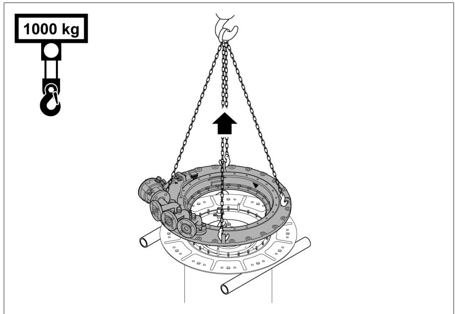
그림 169: 부하시 탭 절환장치 헤드 상단
