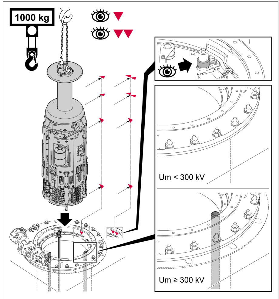
그림 206: 다이버터 스위치 장착부 및 부하시 탭 절환장치 헤드의 표시
