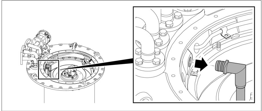
그림 34: 오일 흡입 파이프
