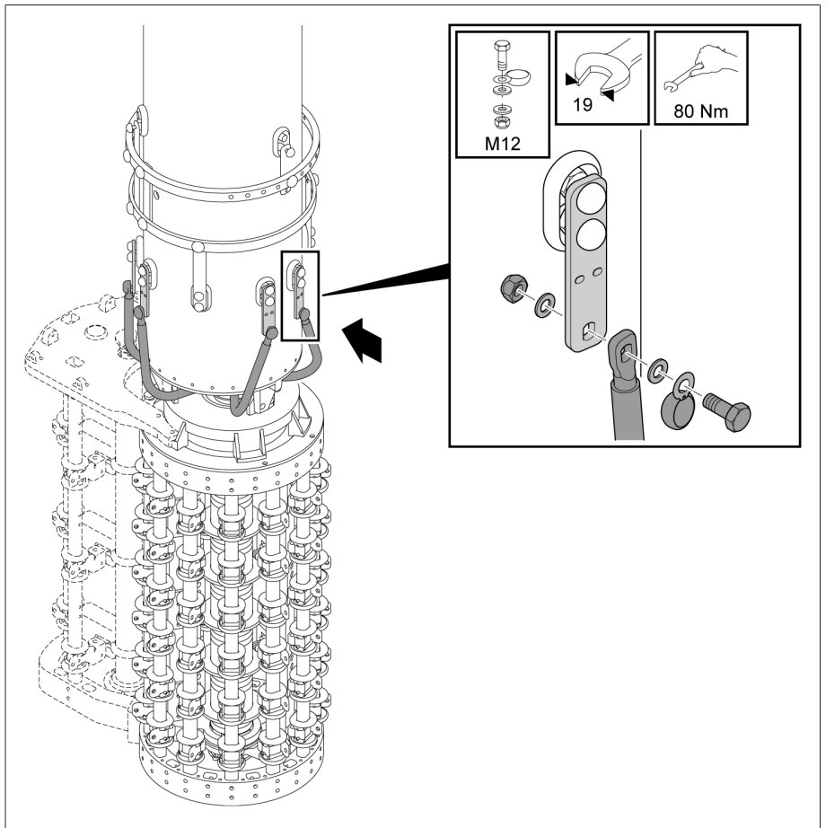
그림 132: 탭 선택기 연결 리드
