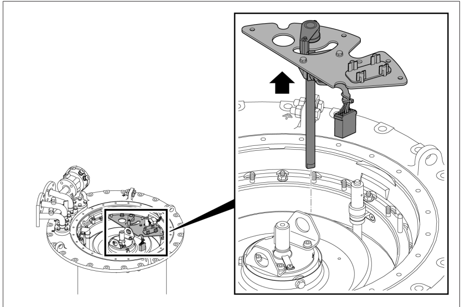
그림 29: 탭 변환 감시 장치 및 구동축과 마운팅 플레이트
