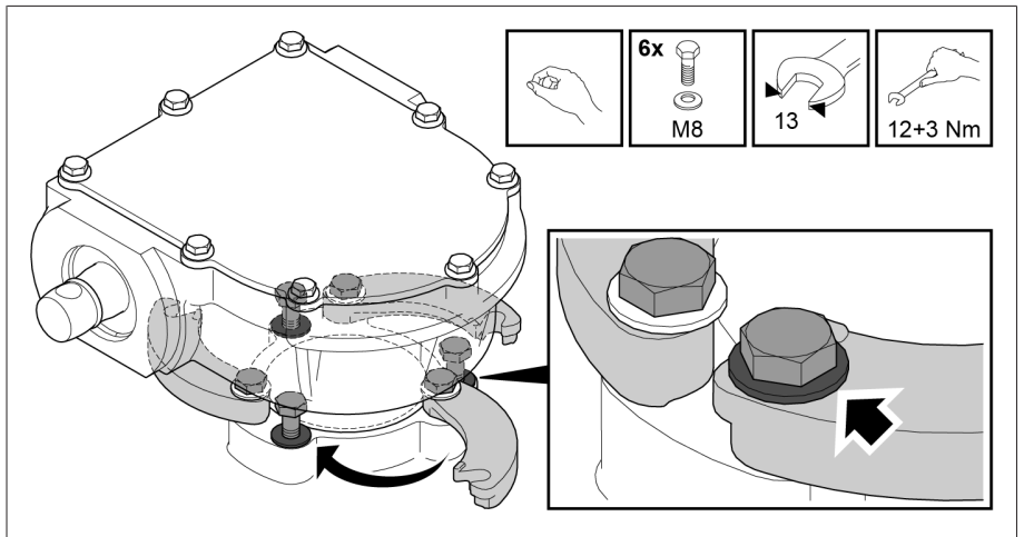
그림 258: 압박 링 세그먼트 고정하기
