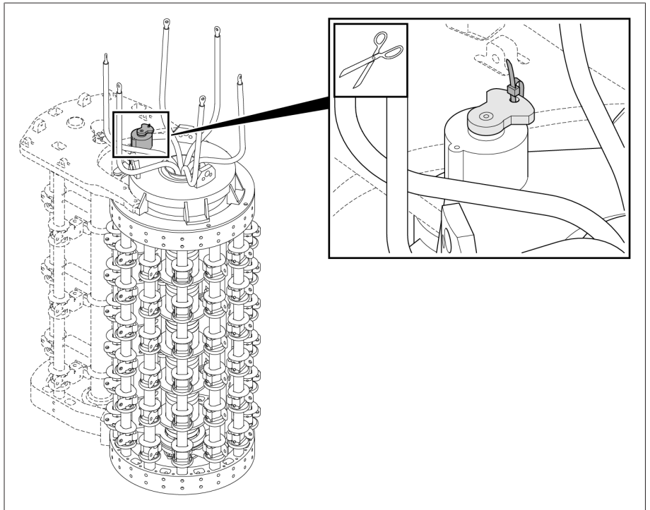
그림 68: 잠금 밴드가 있는 탭 선택기 커플링
