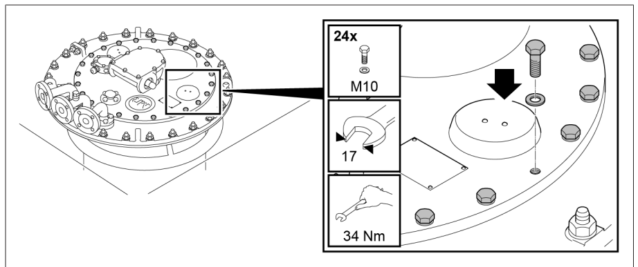
그림 92: 부하시 탭 절환장치 헤드 커버
