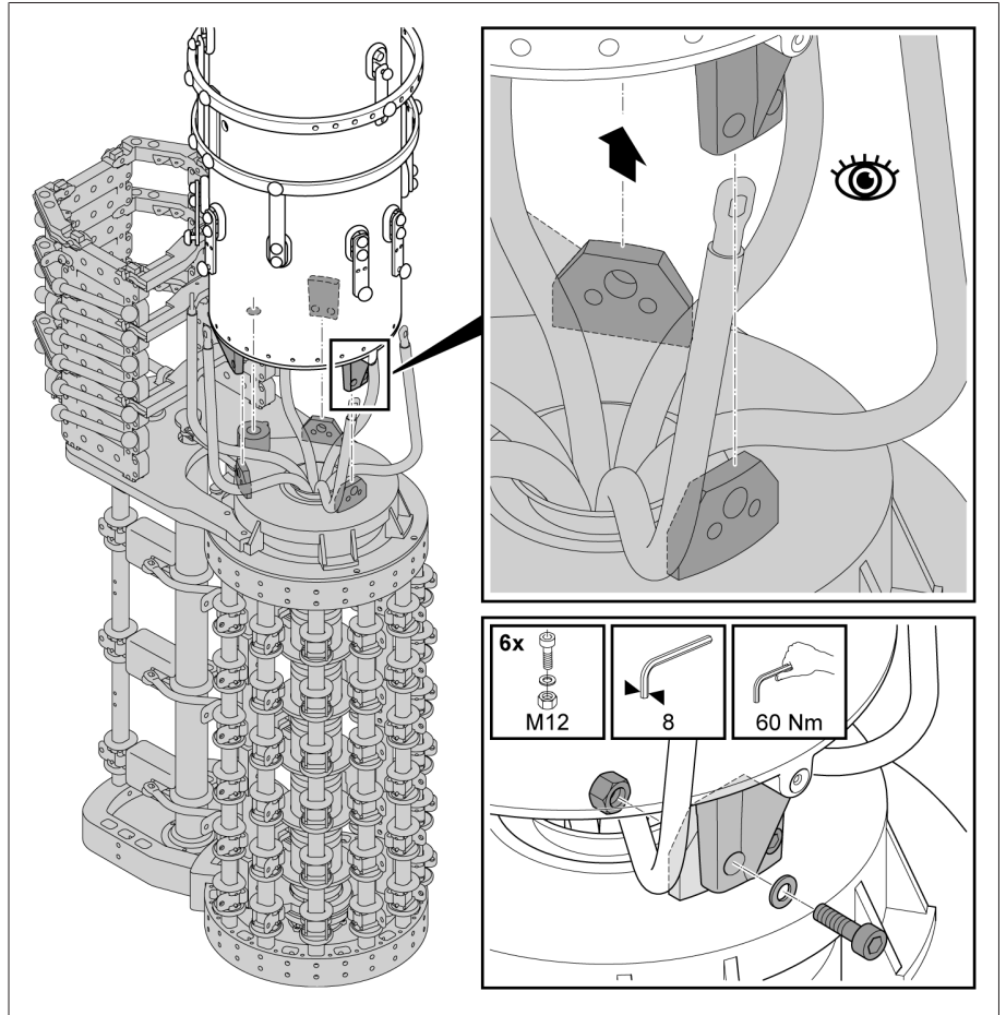
그림 131: 선택기를 유격실에 나사로 고정하기
