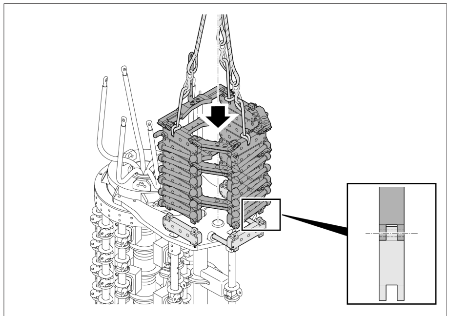
그림 121: 전위연결 기구 내리기
