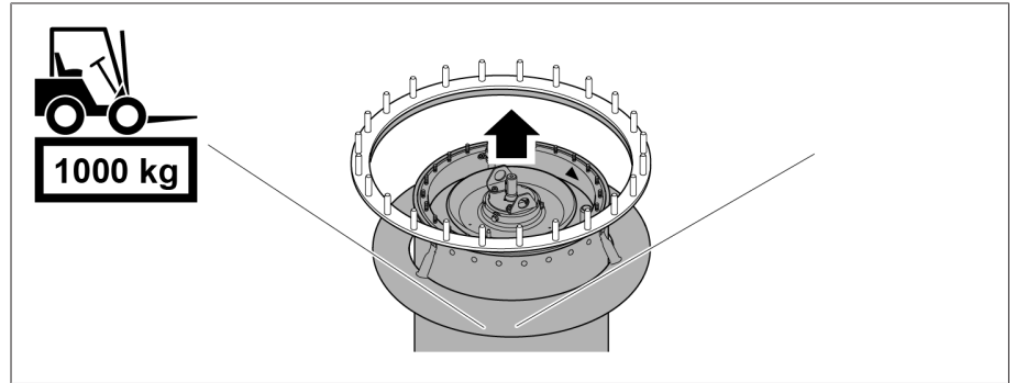
그림 39: 유격실 들어 올리기
