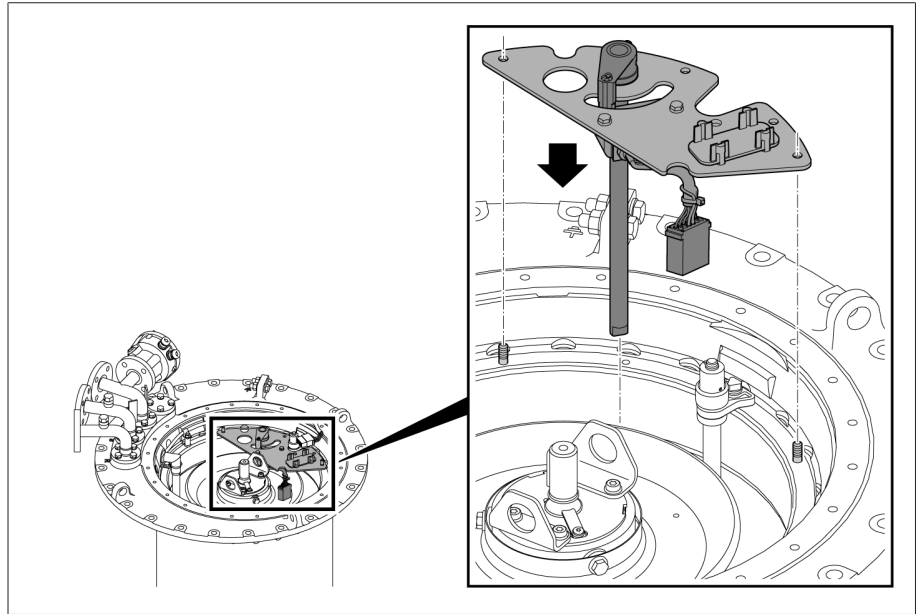
그림 208: 탭 변환 감시 장치 및 구동축과 마운팅 플레이트
