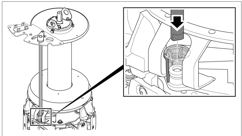
그림 183: 구동축 및 플러그 커넥터
