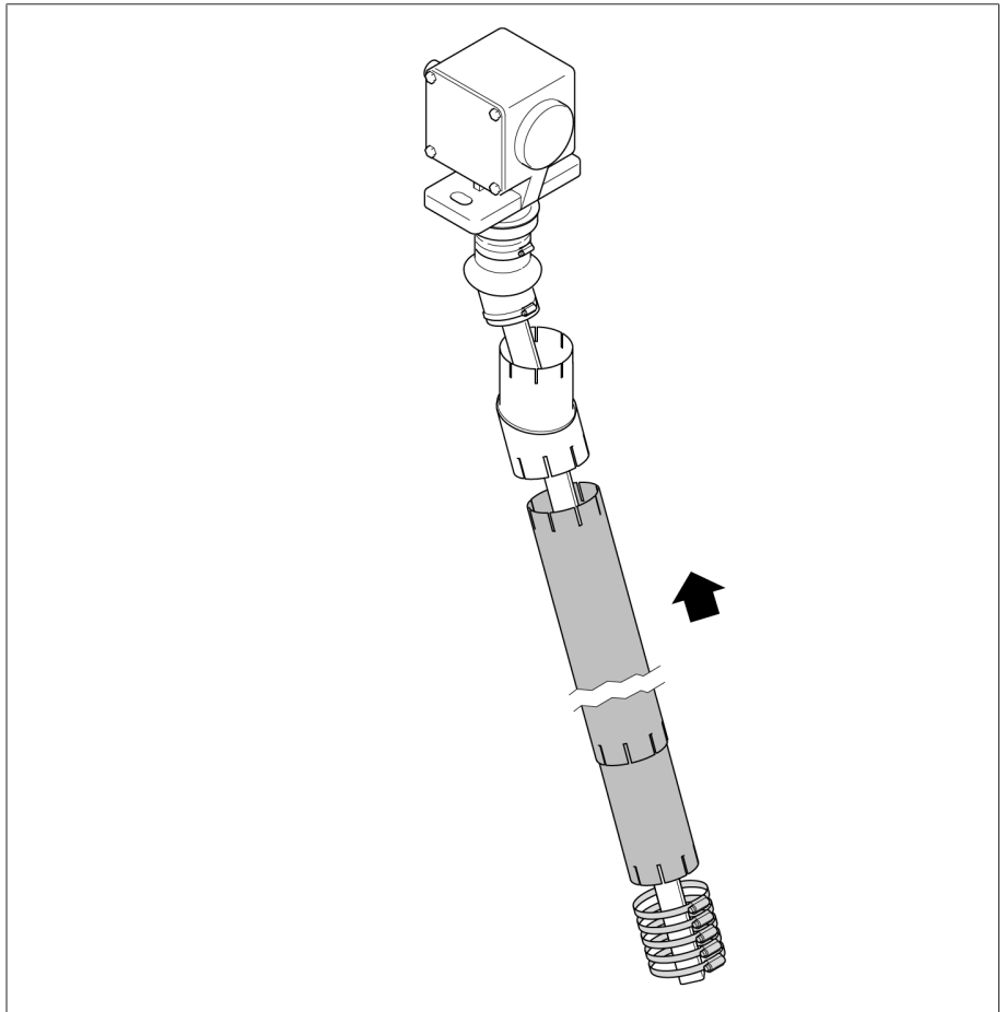
그림 290: 신축 튜브 끼우기
