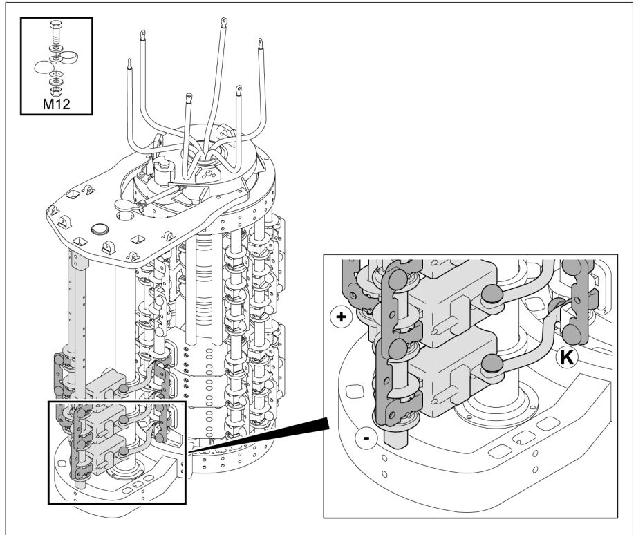
그림 140: 리버싱 체인지 오버 선택기 결선용 체인지 오버 선택기 연결 접점
