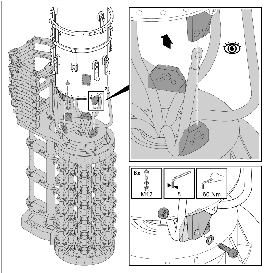
그림 71: 선택기를 유격실에 나사로 고정하기
