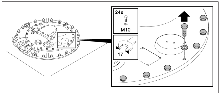
그림 94: 부하시 탭 절환장치 헤드 커버
