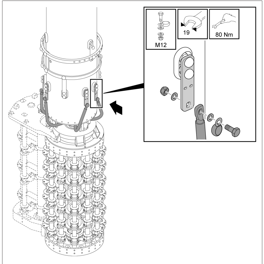
그림 72: 탭 선택기 연결 리드
