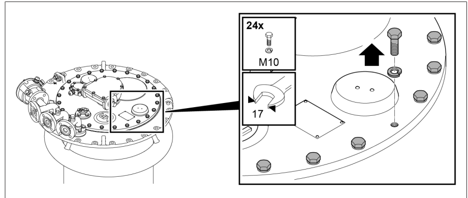
그림 24: 부하시 탭 절환장치 헤드 커버
