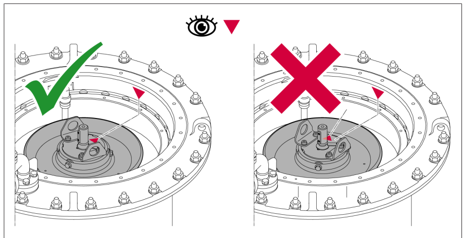
그림 101: 연결 튜브 정렬하기
