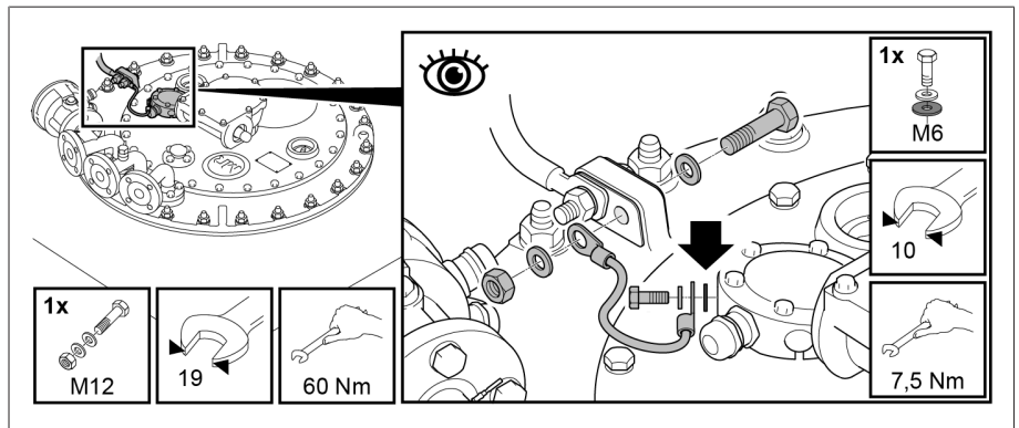
그림 318: 온도 센서 접지하기
