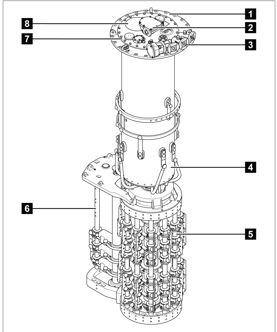
그림 2: 부하시 탭 절환장치 디자인
