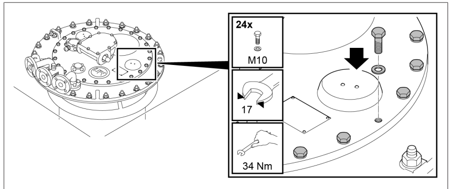
그림 154: 부하시 탭 절환장치 헤드 커버
