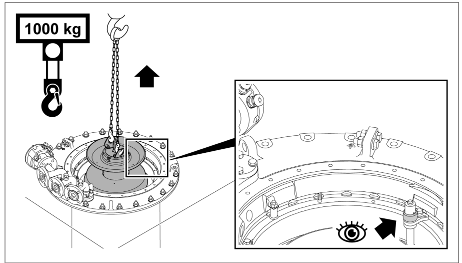
그림 202: 다이버터 스위치 장착부
