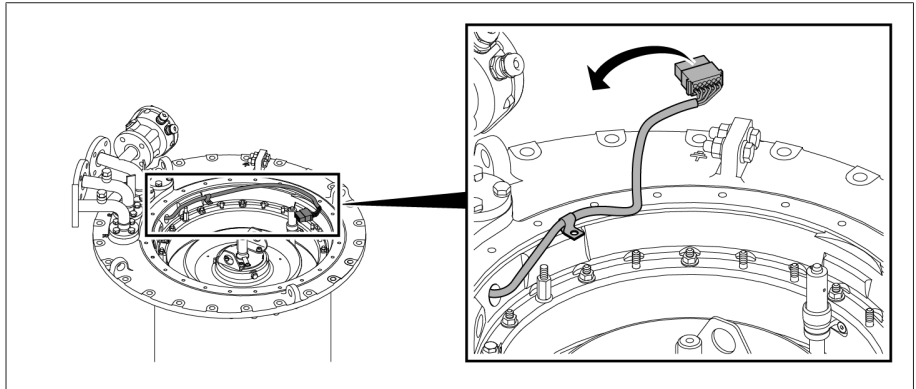
그림 163: 탭 변환 감시 장치의 케이블
