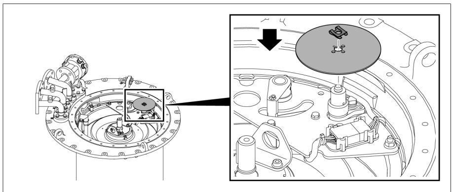
그림 213: 위치 표시 디스크
