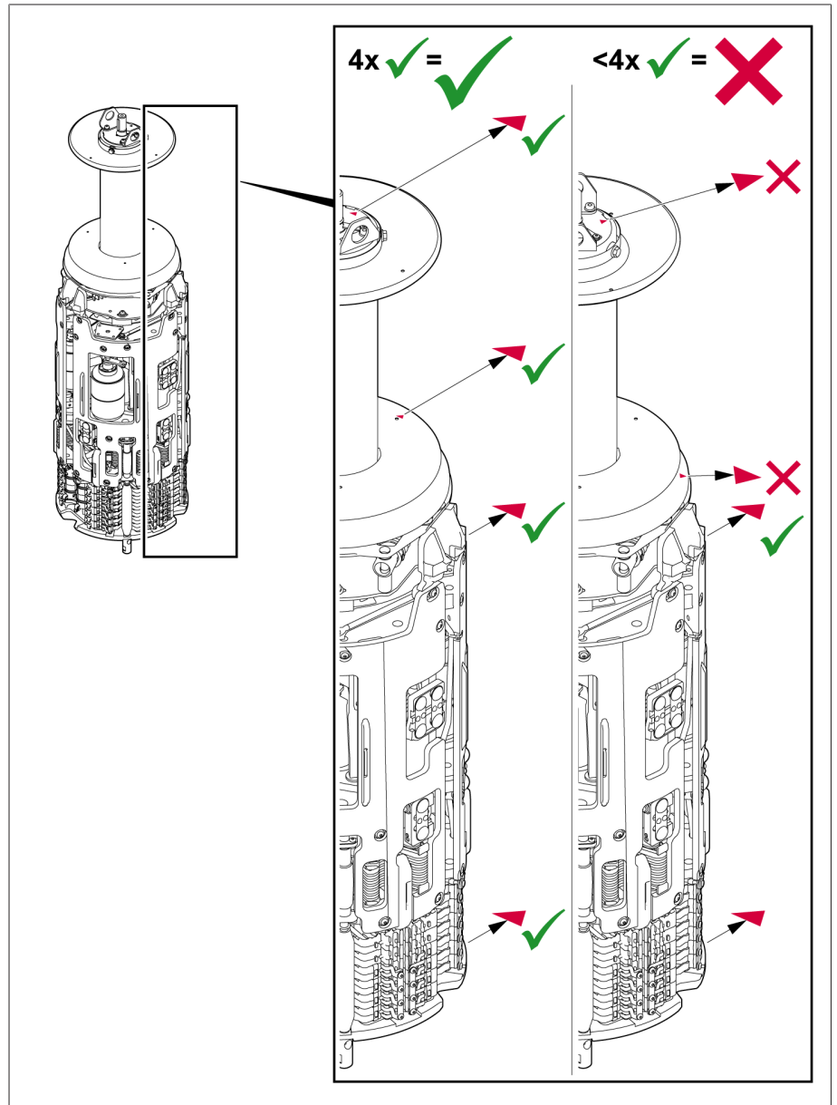
그림 205: 다이버터 스위치 장착부의 표시
