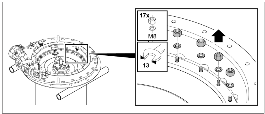
그림 168: 너트가 있는 부하시 탭 절환장치 헤드 상단
