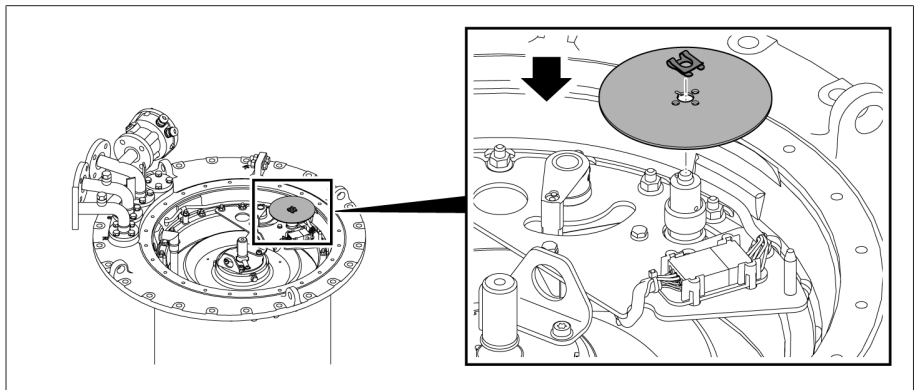
그림 57: 위치 표시 디스크
