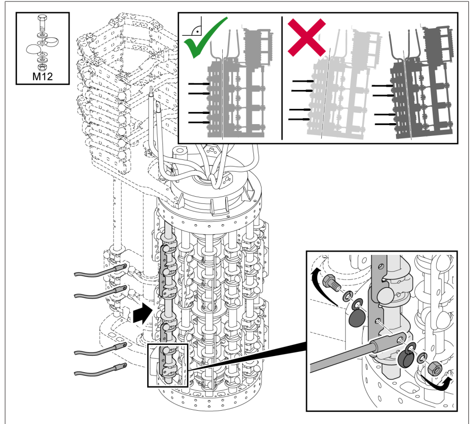
그림 138: 탭 선택기 연결 접점
