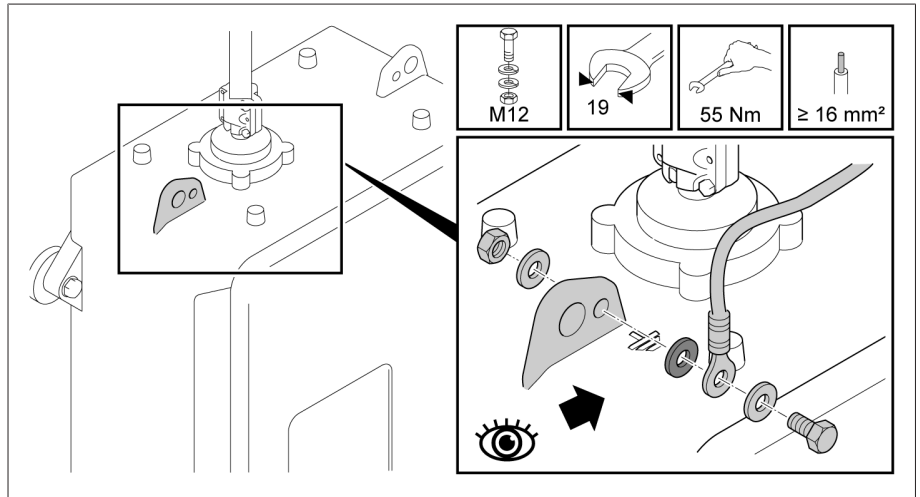
그림 317: 모터 구동 장치 상의 접지 나사
