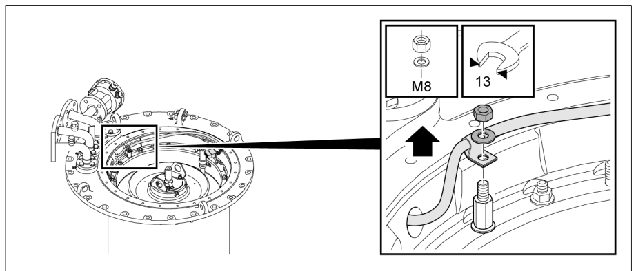
그림 162: 스페이스 볼트와 탭 변환 감시 장치 케이블
