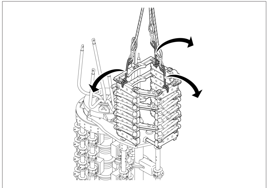
그림 64: 리프팅 스트랩 제거하기
