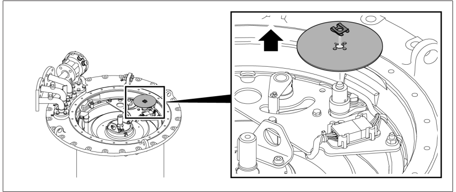
그림 96: 위치 표시 디스크
