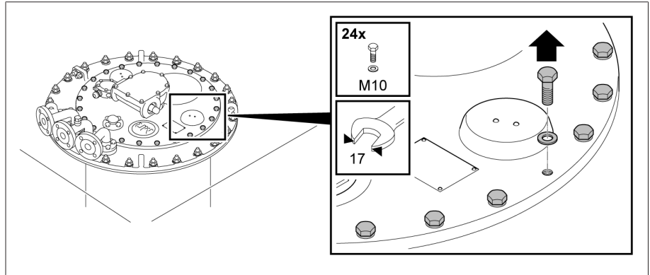
그림 144: 부하시 탭 절환장치 헤드 커버
