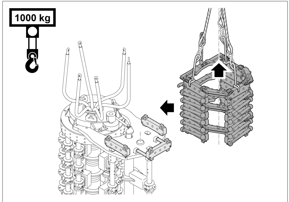
그림 120: 전위연결 기구 들어 올리기
