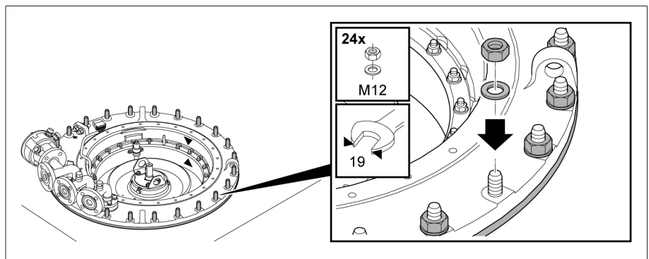
그림 45: 부하시 탭 절환장치 헤드를 마운팅 플랜지에 나사로 고정하기
