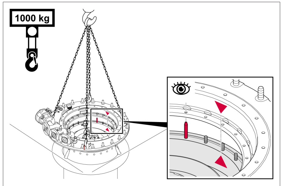
그림 40: 표시와 정렬 핀
