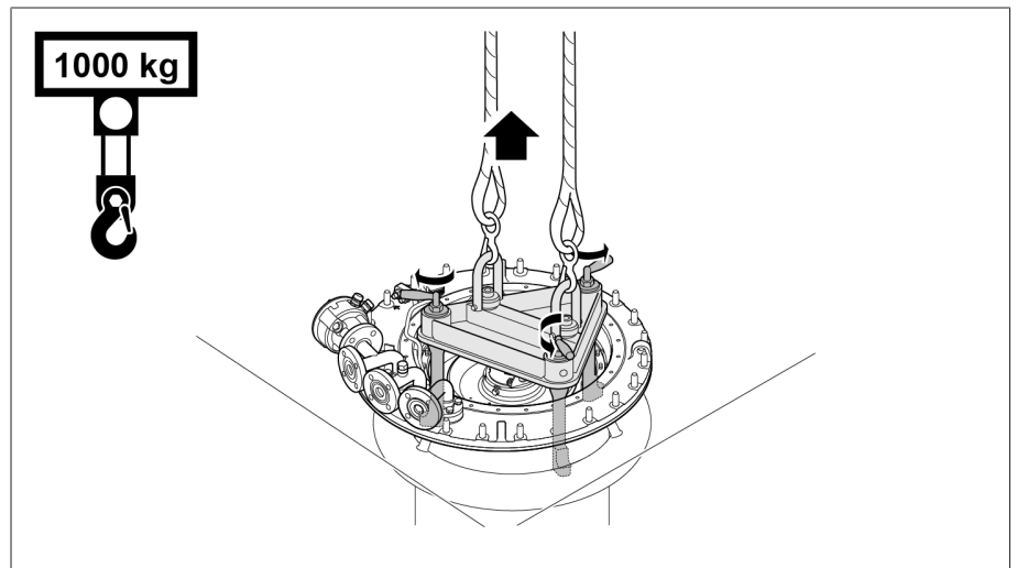
그림 42: 부하시 탭 절환장치 들어 올리기
