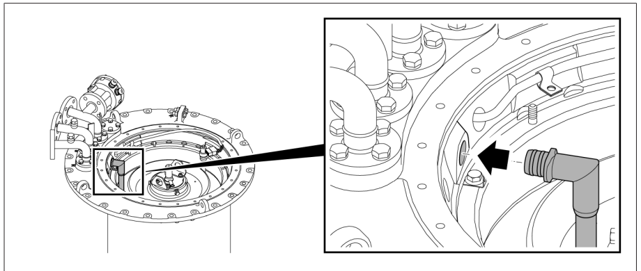
그림 48: 오일 흡입 파이프 끼우기
