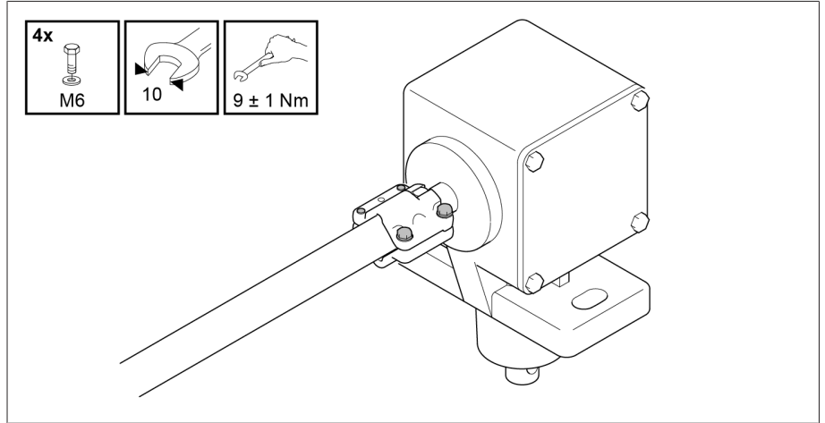
그림 263: 사각 관을 베벨 기어에 고정하기
