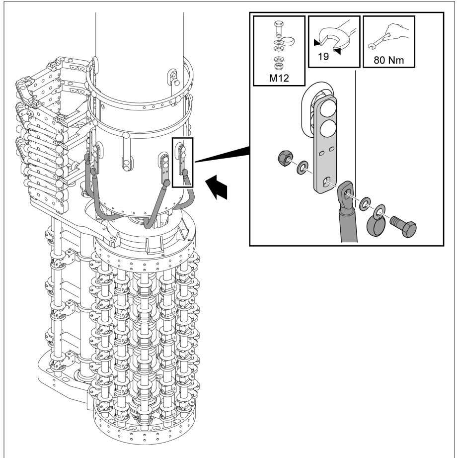
그림 73: 탭 선택기 연결 리드
