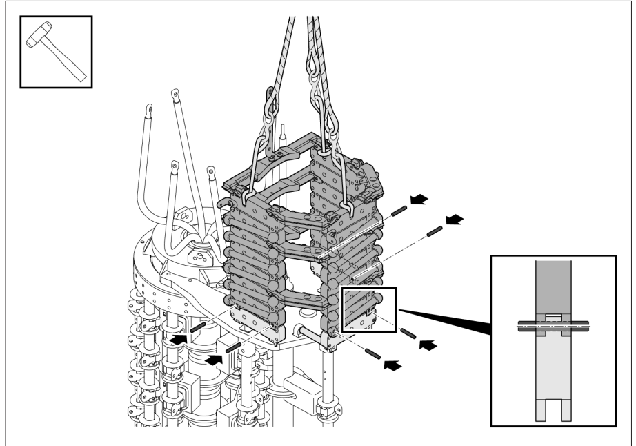
그림 63: 전위연결 기구 고정
