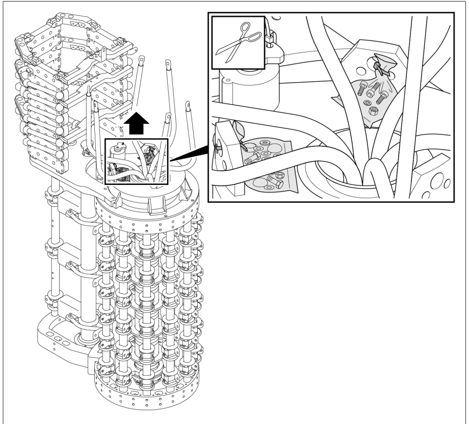
그림 126: 체결 부품이 들어 있는 비닐봉지
