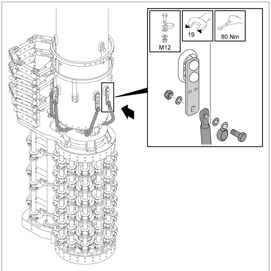
그림 133: 탭 선택기 연결 리드
