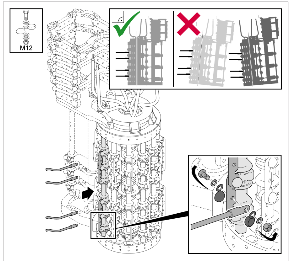
그림 76: 탭 선택기 연결 접점
