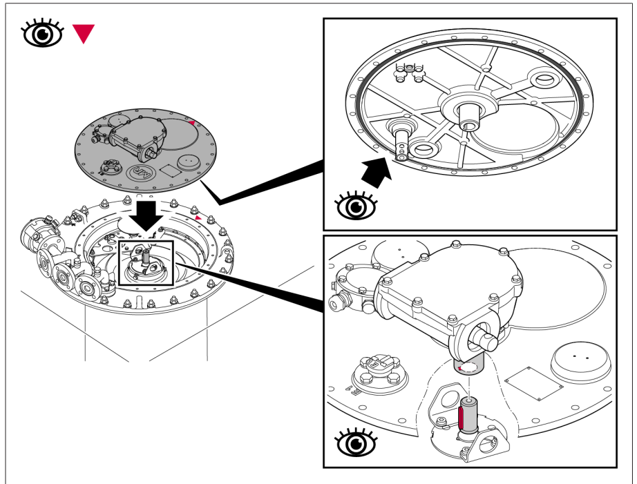
그림 91: O-링이 있는 부하시 탭 절환장치 헤드 커버
