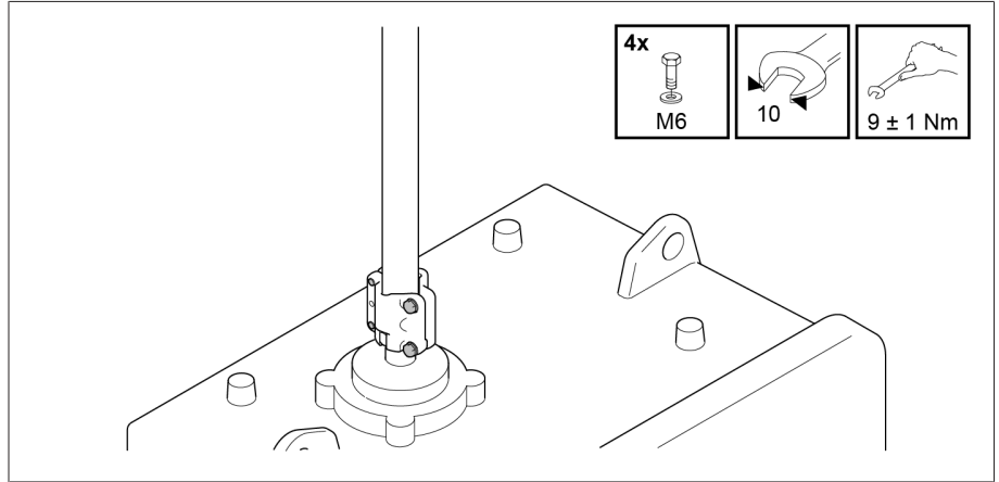
그림 248: 구동 장치에 사각 관 연결하기
