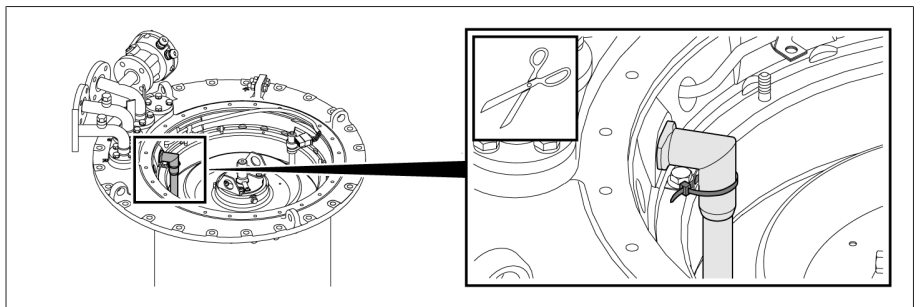
그림 33: 오일 흡입 파이프
