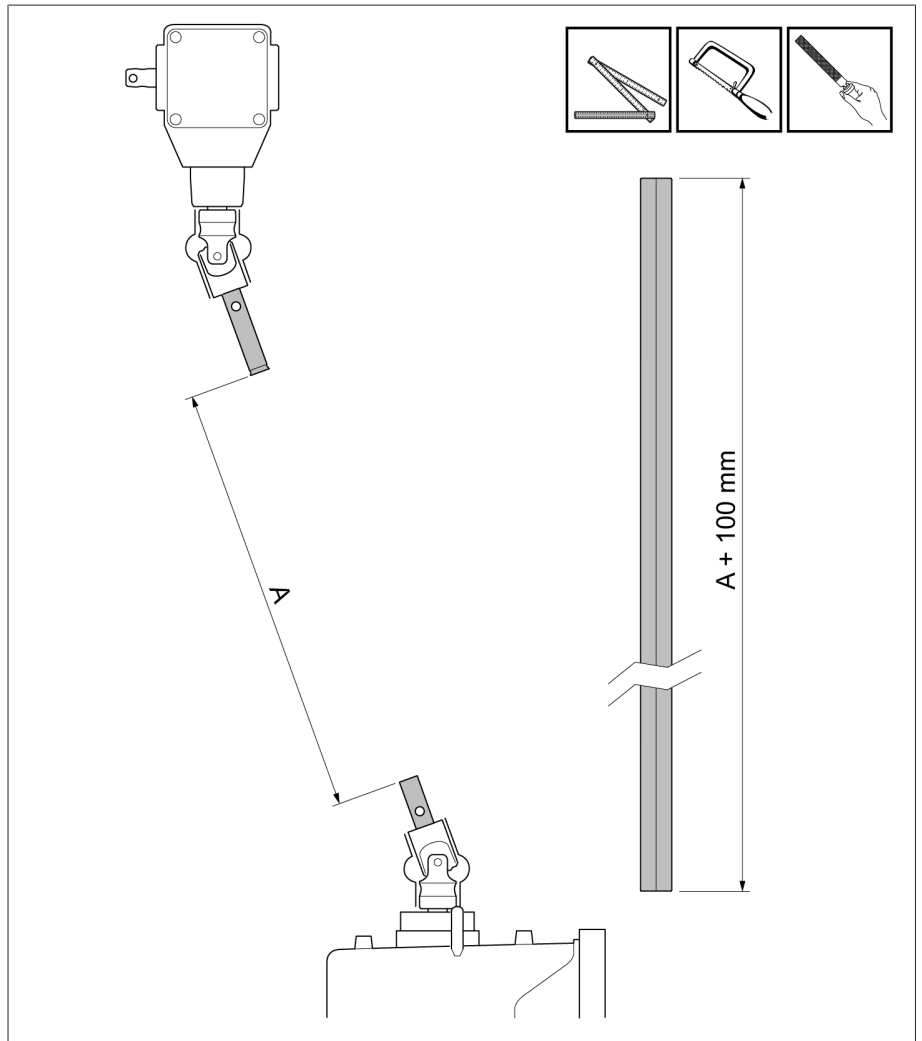
그림 285: 사각 관 줄이기
