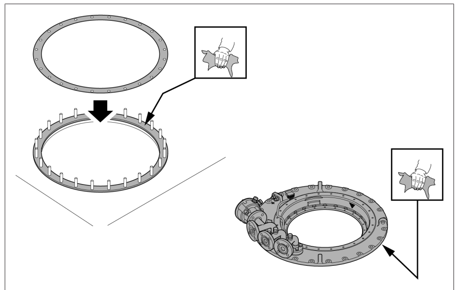
그림 38: 개스킷이 있는 마운팅 플랜지
