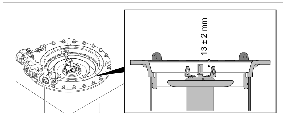
그림 207: 다이버터 스위치 장착부 어댑터 샤프트의 위쪽 가장자리와 부하시 탭 절환장치 헤드 장착면 사이의 거리
