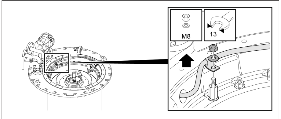
그림 30: 스페이스 볼트와 탭 변환 감시 장치 케이블
