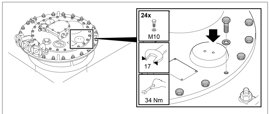
그림 60: 부하시 탭 절환장치 헤드 커버
