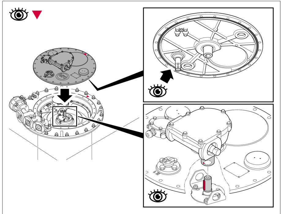
그림 215: O-링이 있는 부하시 탭 절환장치 헤드 커버
