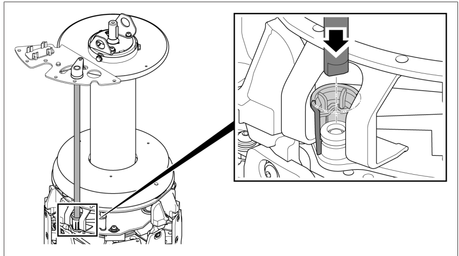
그림 109: 구동축 및 플러그 커넥터
