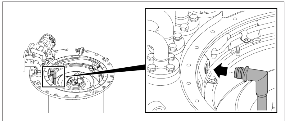
그림 180: 오일 흡입 파이프 끼우기
