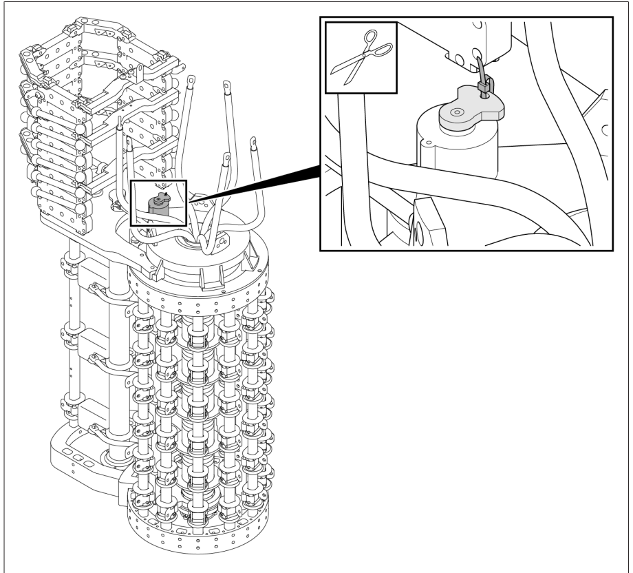
그림 128: 잠금 밴드가 있는 탭 선택기 커플링
