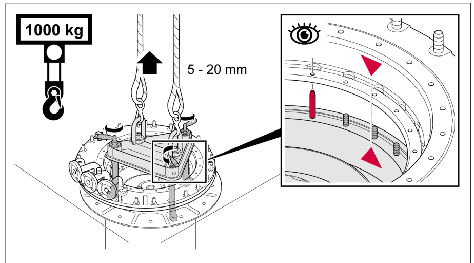
그림 175: 부하시 탭 절환장치 들어 올리기
