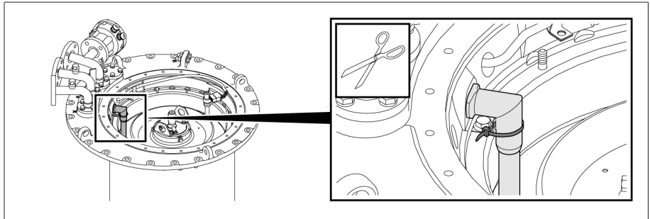
그림 165: 오일 흡입 파이프
