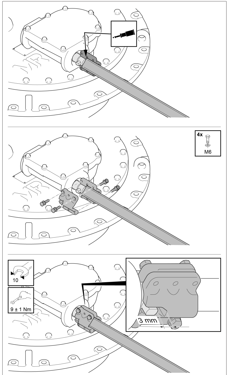
그림 264: 사각 관을 상부 기어 유닛에 고정합니다.
