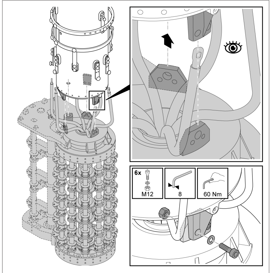
그림 130: 선택기를 유격실에 나사로 고정하기
