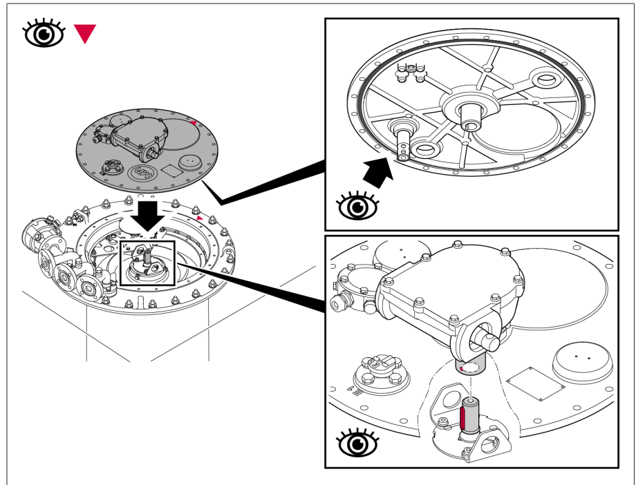
그림 191: O-링이 있는 부하시 탭 절환장치 헤드 커버
