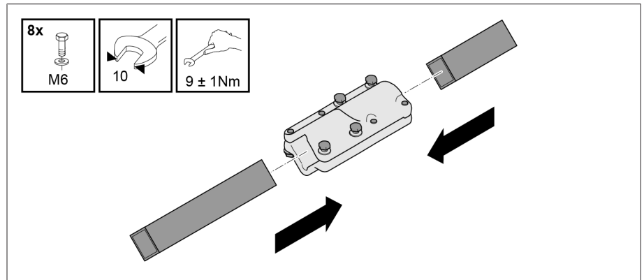
그림 301: 이중 연결 부품을 사용하여 사각 관 및 절연체를 나사로 조입니다.
