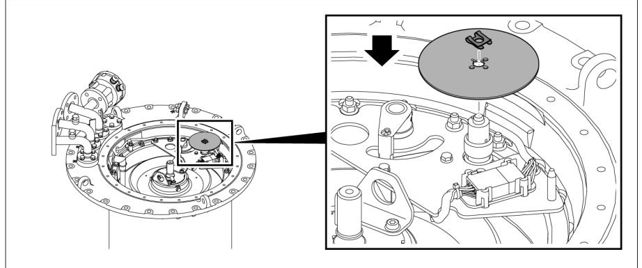
그림 189: 위치 표시 디스크
