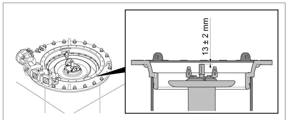
그림 107: 다이버터 스위치 장착부 어댑터 샤프트의 위쪽 가장자리와 부하시 탭 절환장치 헤드 장착면 사이의 거리
