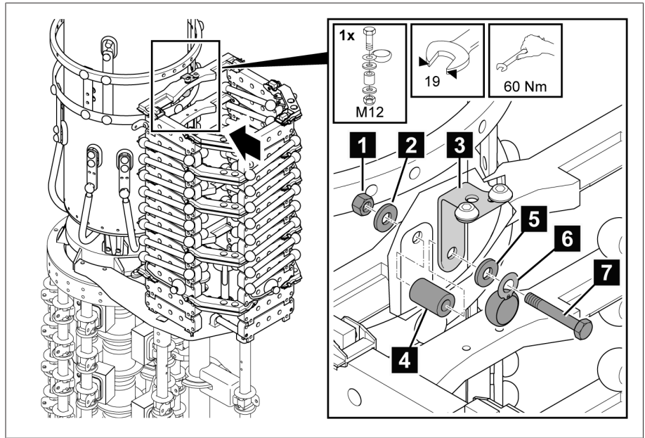
그림 75: 전위연결 기구 고정
