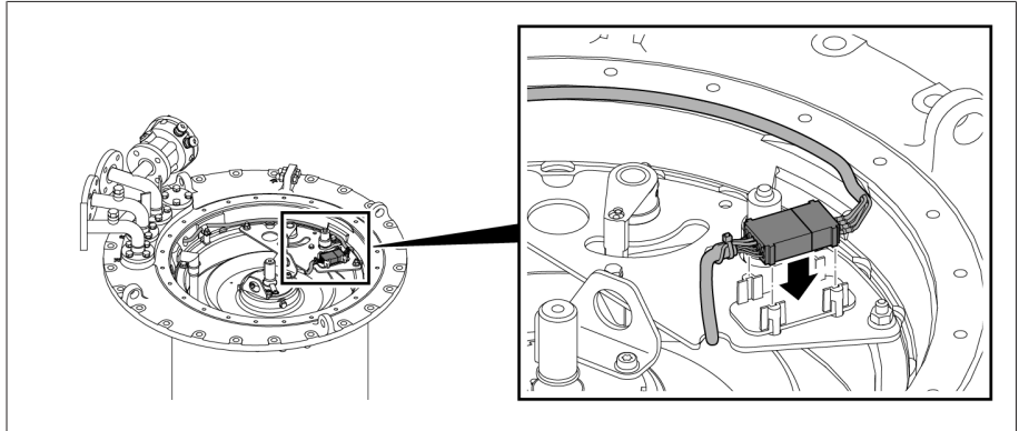
그림 56: 브래킷에 끼운 플러그 커넥터
