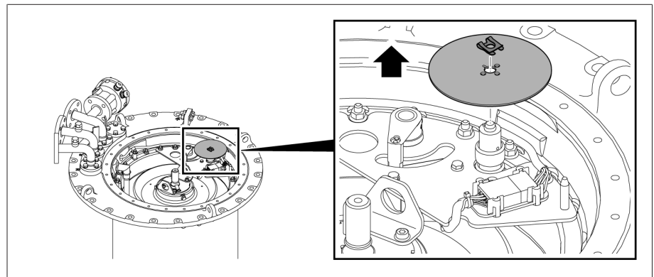
그림 26: 위치 표시 디스크
