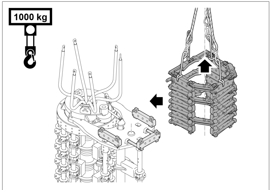
그림 61: 전위연결 기구 들어 올리기
