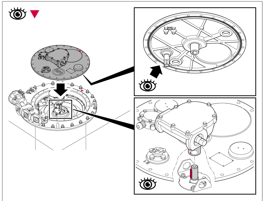
그림 147: O-링이 있는 부하시 탭 절환장치 헤드 커버
