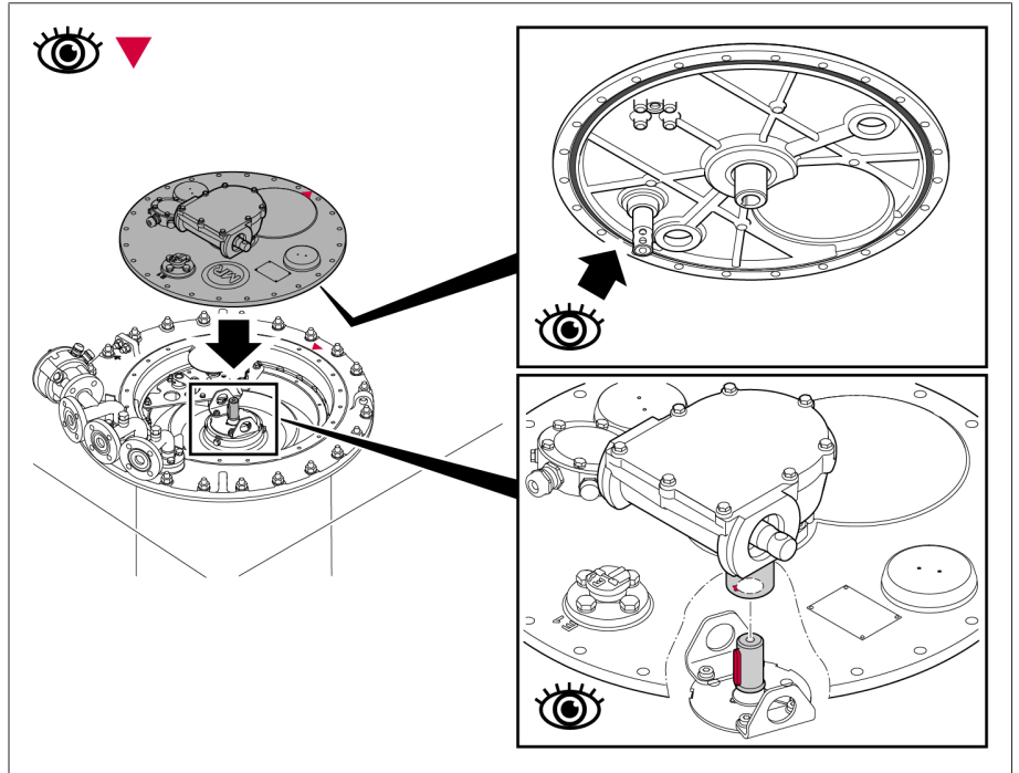
그림 153: O-링이 있는 부하시 탭 절환장치 헤드 커버
