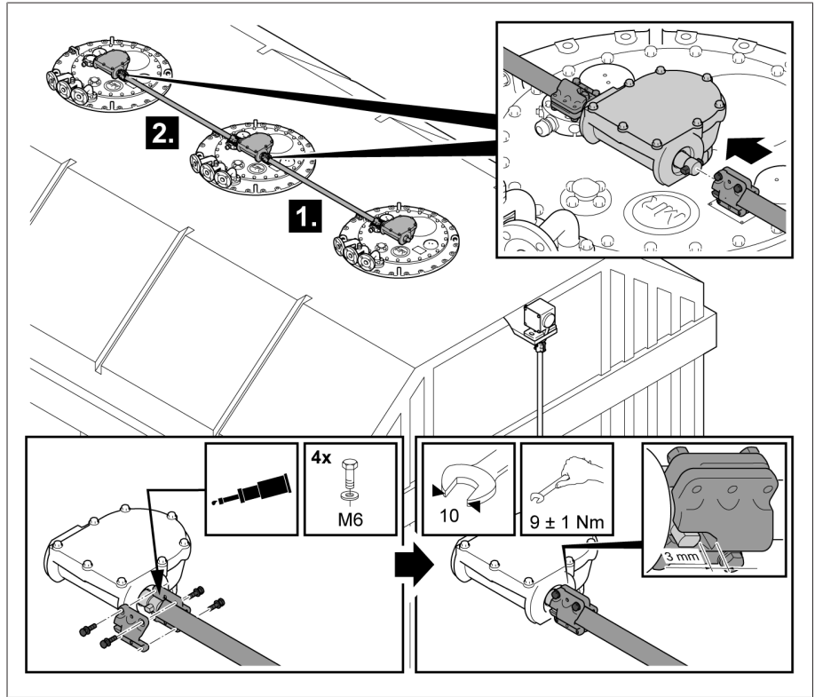
그림 272: 부하시 탭 절환장치 컬럼 연결하기
