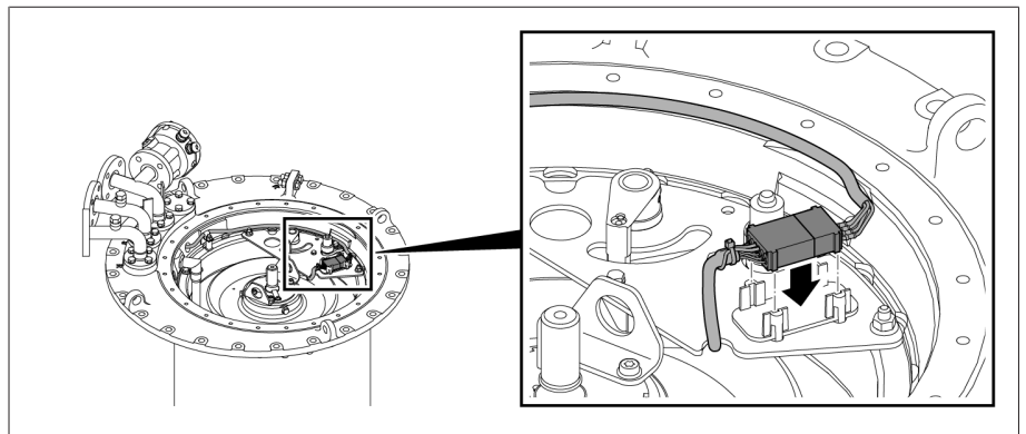
그림 188: 브래킷에 끼운 플러그 커넥터
