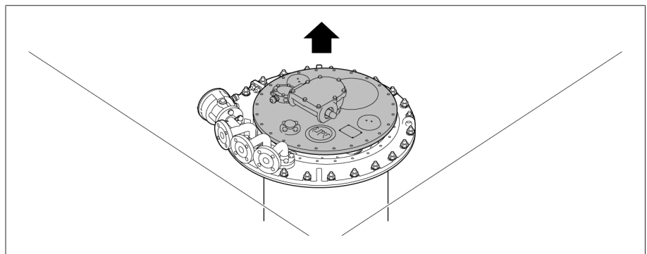
그림 95: 부하시 탭 절환장치 헤드 커버
