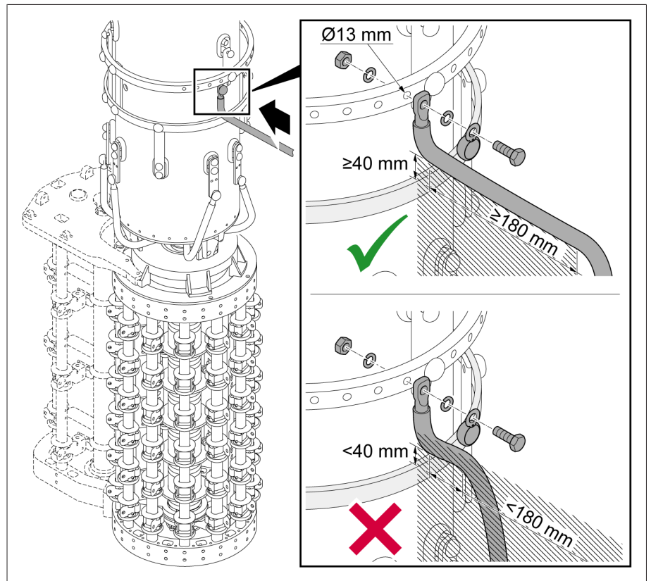
그림 143: 유격실의 인출 링
