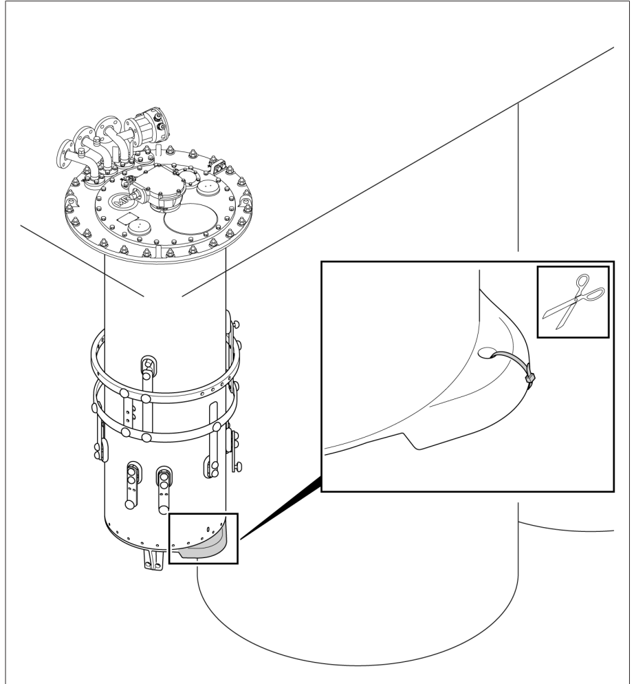
그림 23: 잠금 밴드가 있는 유격실 하부
