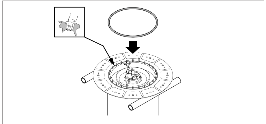
그림 170: O-링이 있는 지지플랜지
