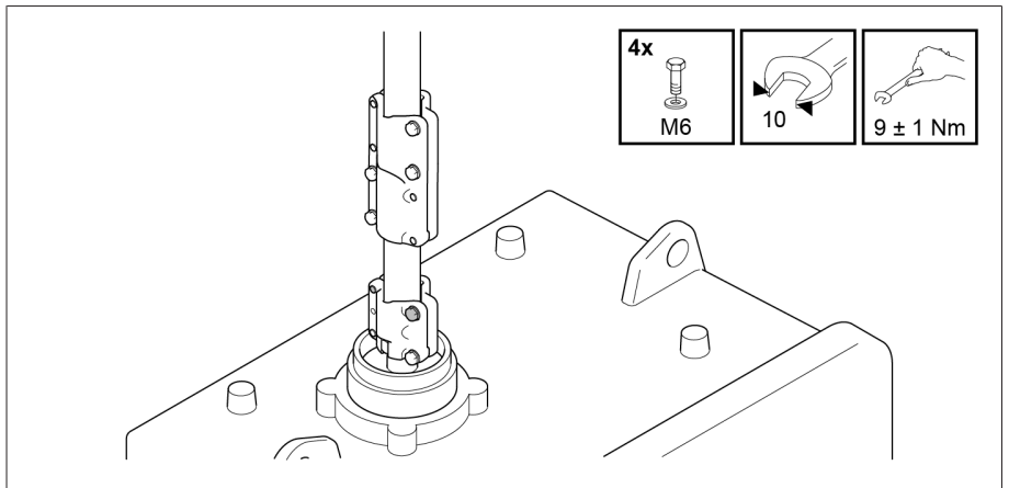
그림 305: 구동 장치에 사각 관 연결하기
